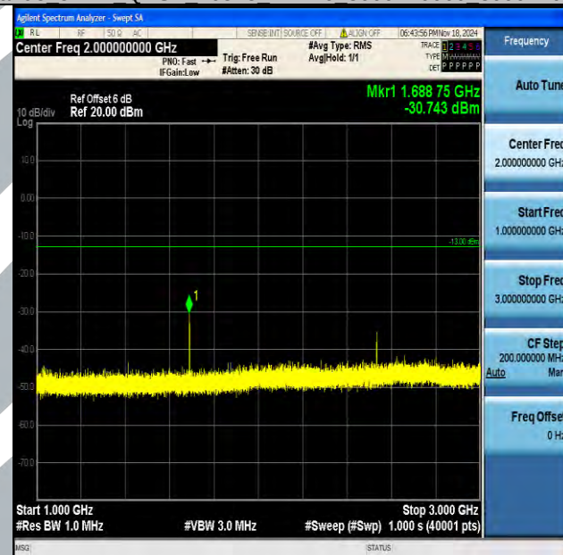
Band5 5MHz QPSK 20625 1RB#0 1000~3000 1000~3000
