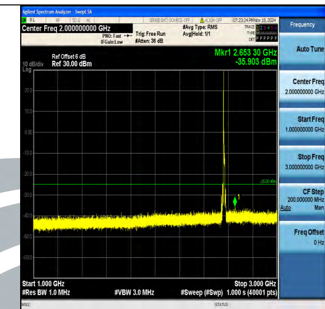
Band7 10MHz 16QAM 21400 1RB#0 1000~3000 1000~3000
