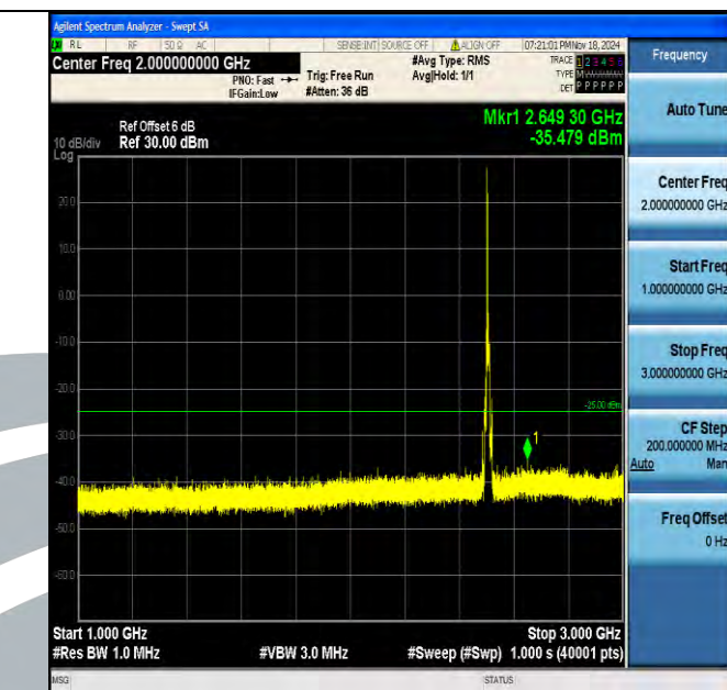
Band7 10MHz 16QAM 20800 1RB#0 1000~3000 1000~3000
