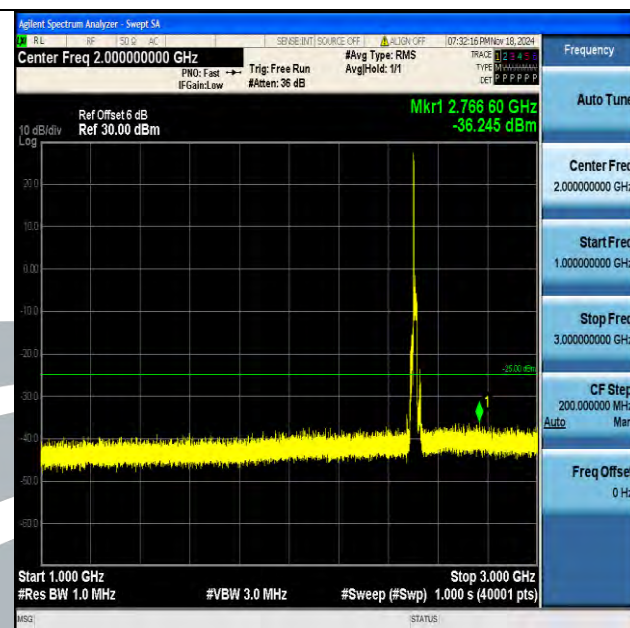
Band7 15MHz 16QAM 20825 1RB#0 1000~3000 1000~3000
