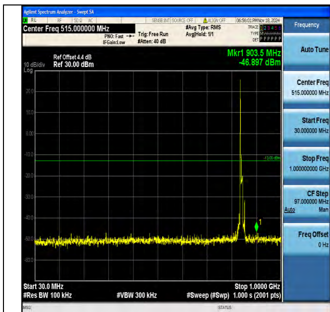
Band5 10MHz QPSK 20600 1RB#0 30~1000 30~1000
