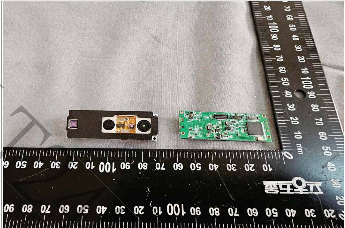
< PCB6-F >
