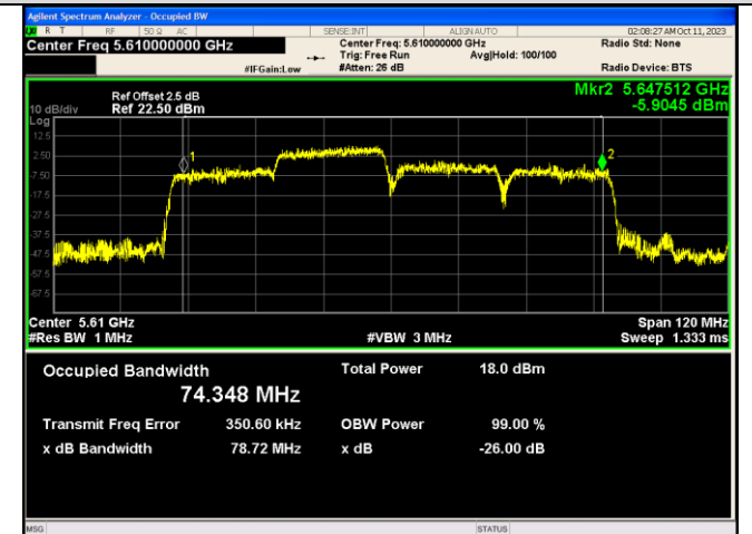
IEEE 802.11ax_Channel 122_80MHz_Antenna 1_RU&Index 242RU62
