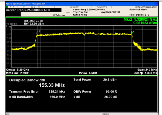
IEEE 802.11ax_Channel 50_160MHz_Antenna 1_RU&Index 996*2RU68
