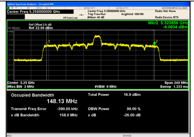
IEEE 802.11ax_Channel 50_160MHz_Antenna 1_RU&Index 106RU60
