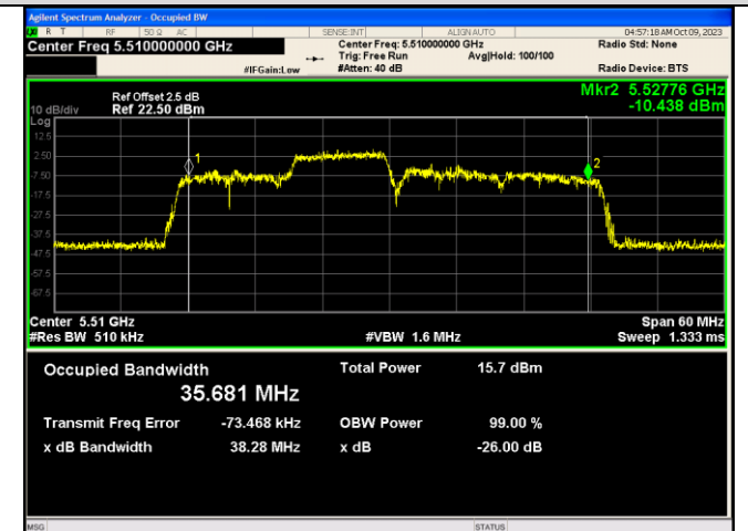
IEEE 802.11ax_Channel 102_40MHz_Antenna 1_RU&Index 106RU54
