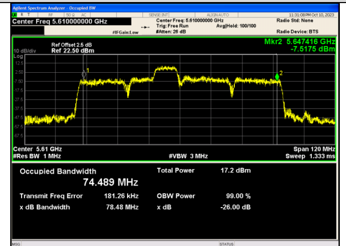
IEEE 802.11ax_Channel 122_80MHz_Antenna 1_RU&Index 106RU56
