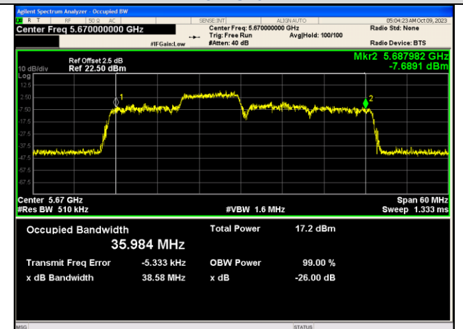
IEEE 802.11ax_Channel 134_40MHz_Antenna 1_RU&Index 106RU54
