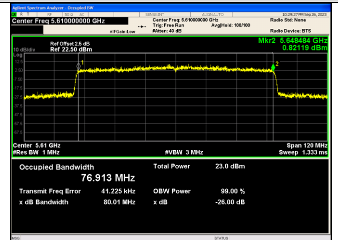
IEEE 802.11ax_Channel 122_80MHz_Antenna 1_RU&Index 996RU67
