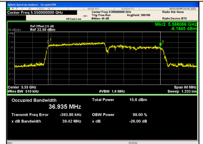
IEEE 802.11ax_Channel 110_40MHz_Antenna 1_RU&Index 242RU61
