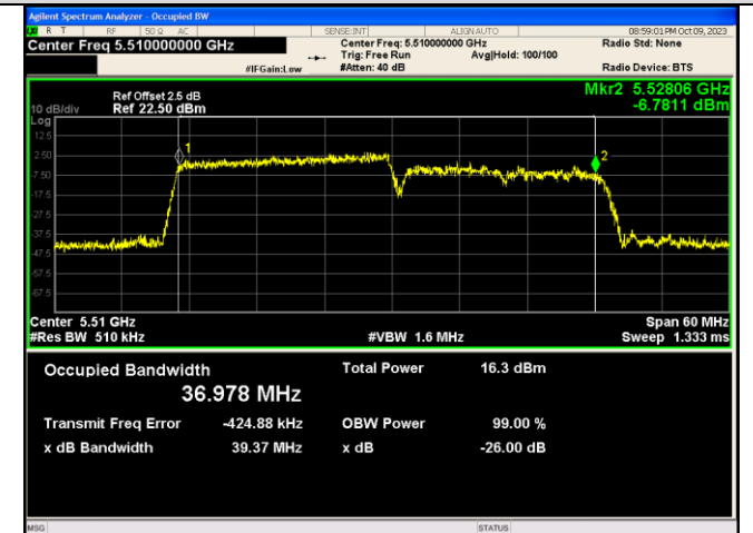
IEEE 802.11ax_Channel 102_40MHz_Antenna 1_RU&Index 242RU61
