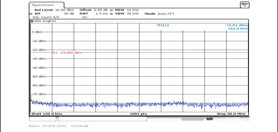
Band13-10MHz-QPSK-23230-1RB#0-Range2:0.15~30MHz-PASS
