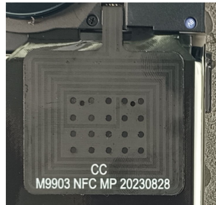
NFC antenna
