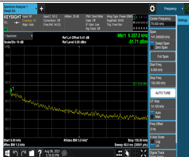
Band2-5MHz-QPSK-18900-1-0-Low-0.009-0.15--51.71-PASS
