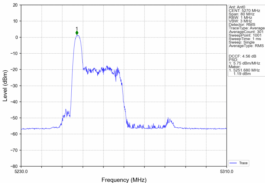
802.11ax(HEW40)_LCH_5270MHz_RU26_Left_Ant0_NTNV
