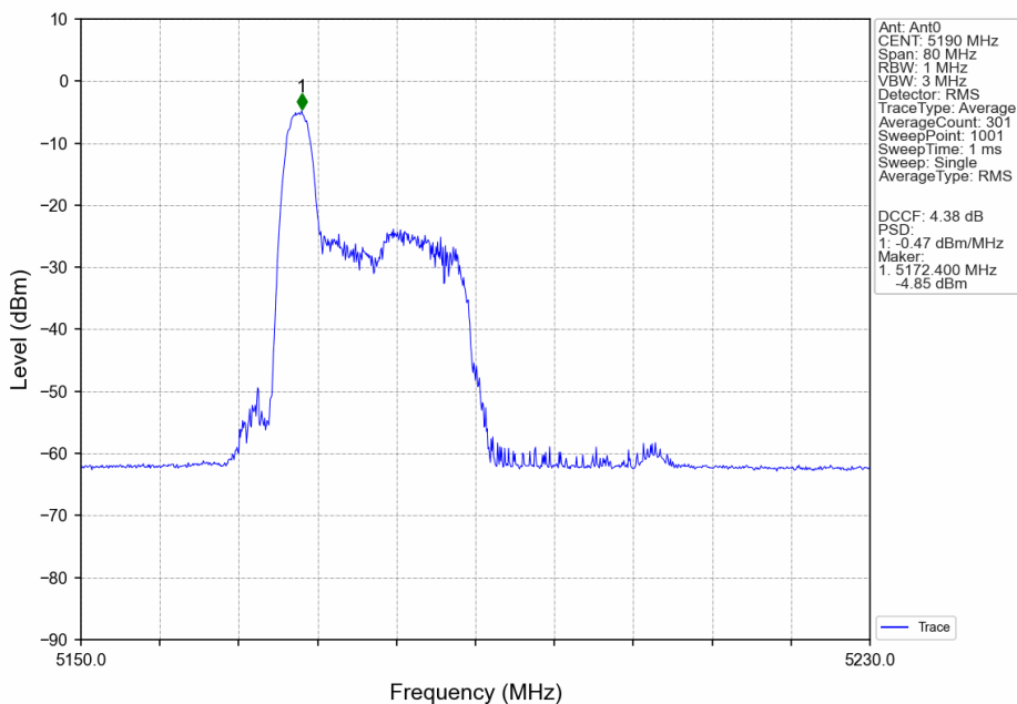
802.11ax(HEW40)_LCH_5190MHz_RU26_Left_Ant0_NTNV
