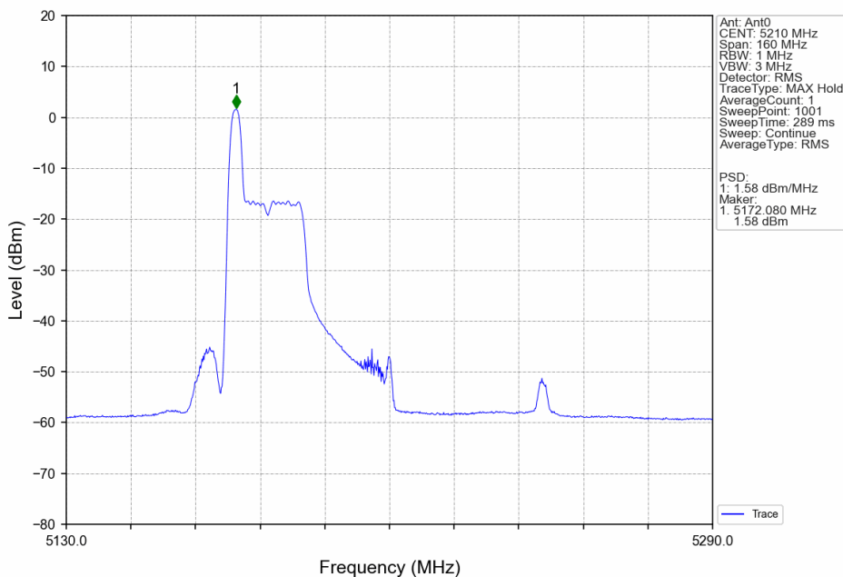
802.11ax(HEW80)_MCH_5210MHz_RU26_Left_Ant0_NTNV
