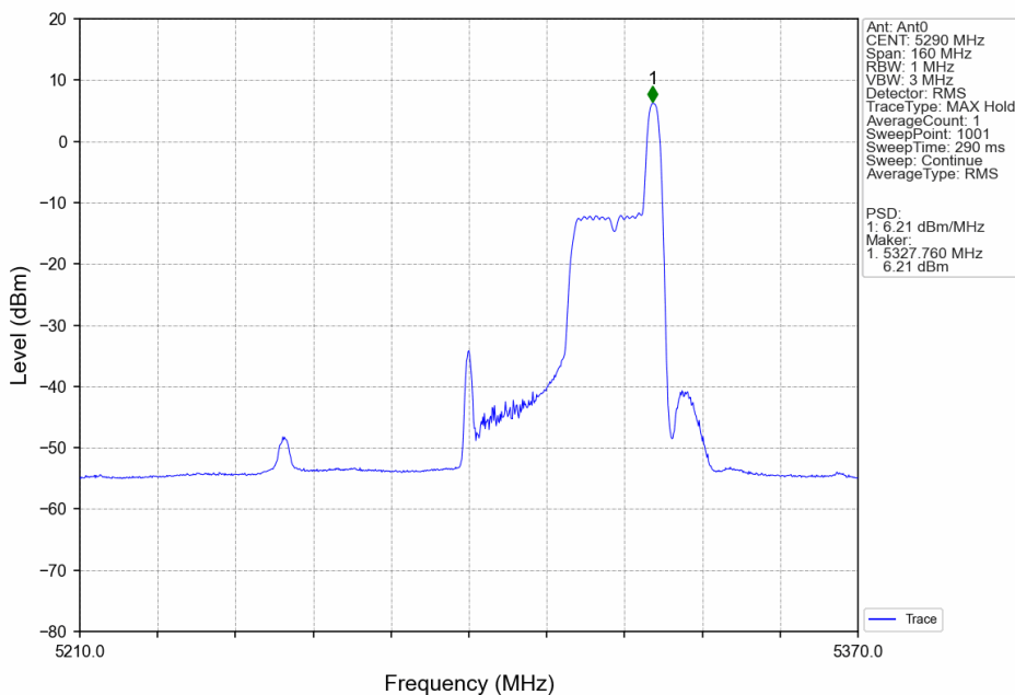
802.11ax(HEW80)_MCH_5290MHz_RU26_Right_Ant0_NTNV
