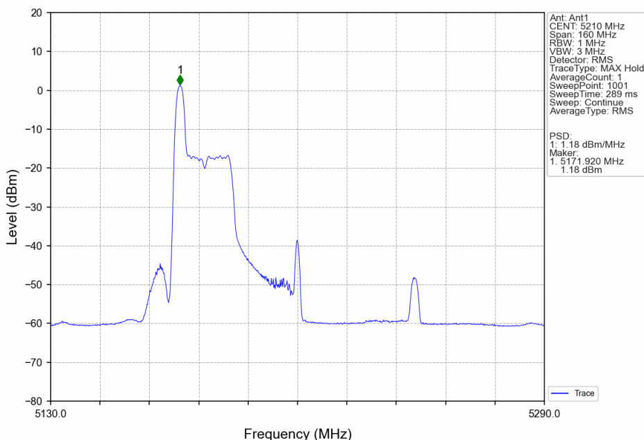
802.11ax(HEW80)_MCH_5210MHz_RU26_Left_MIMO_NTNV
