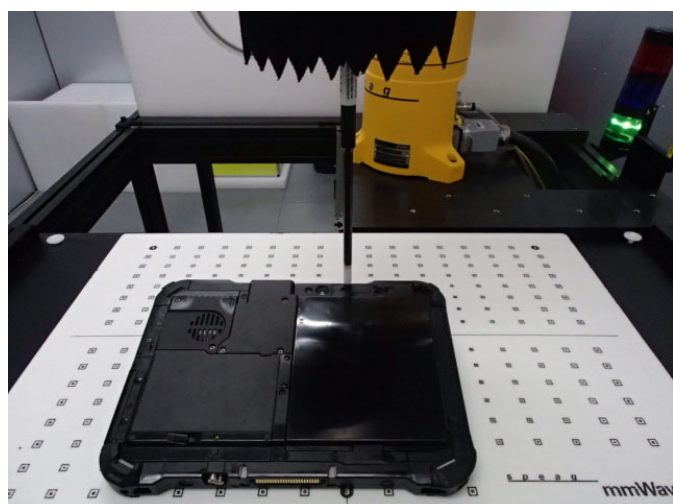
Module #2 (Rear tilt Edge 1 side)
