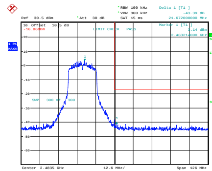
ax20_2462MHz
