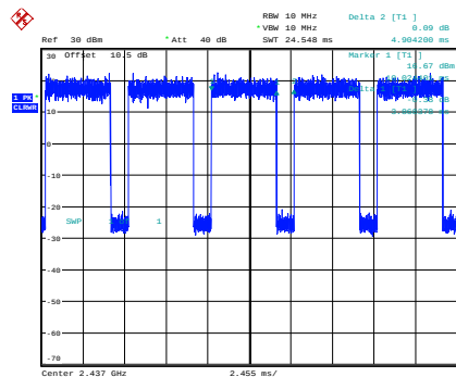
ax20_2437MHz
