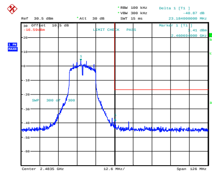
n20_2462MHz
