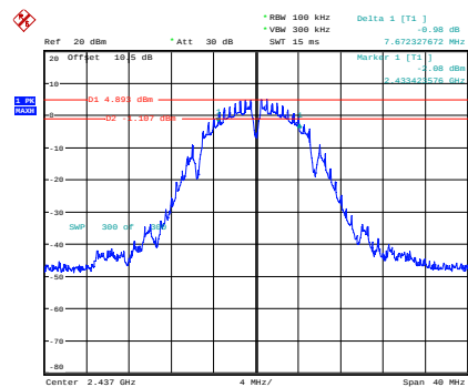
b_2437MHz
