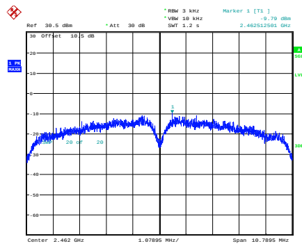
b_2462MHz_Chain 0
