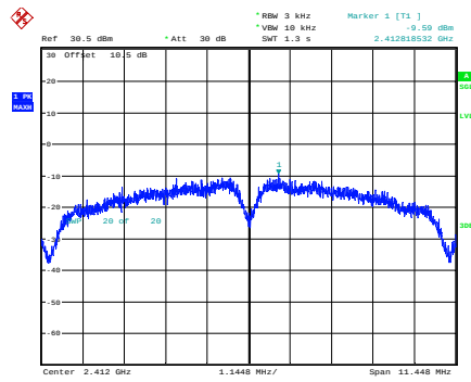
b_2412MHz
