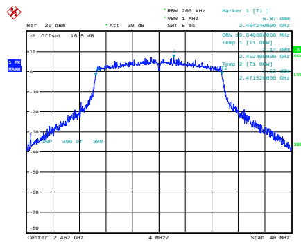
ax20_2462MHz
