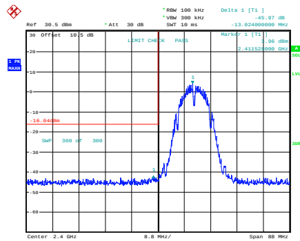
b_2412MHz
