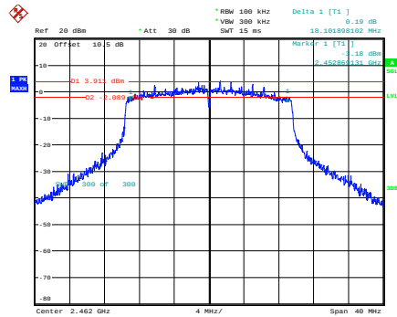
ax20_2462MHz
