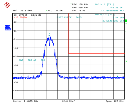
b_2462MHz
