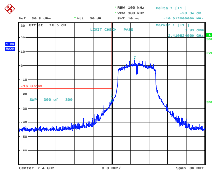
n20_2412MHz
