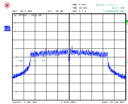
g_2462MHz
