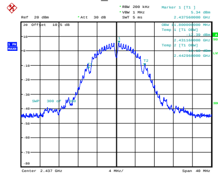
b_2437MHz
