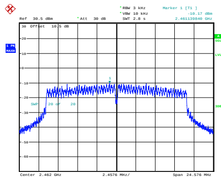
n20_2462MHz
