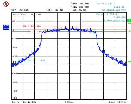
ax20_2412MHz
