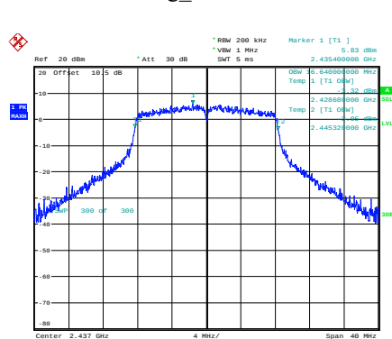
g_2437MHz
