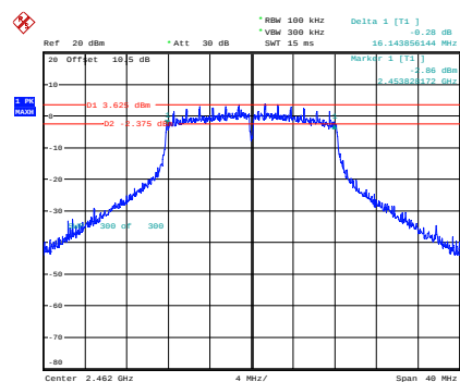
g_2462MHz
