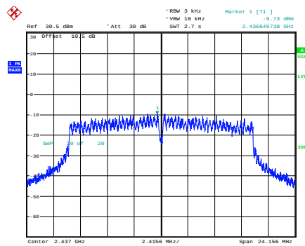
g_2437MHz
