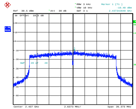
ax20_2437MHz
