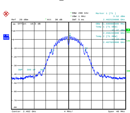
b_2462MHz
