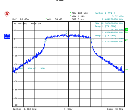
g_2462MHz
