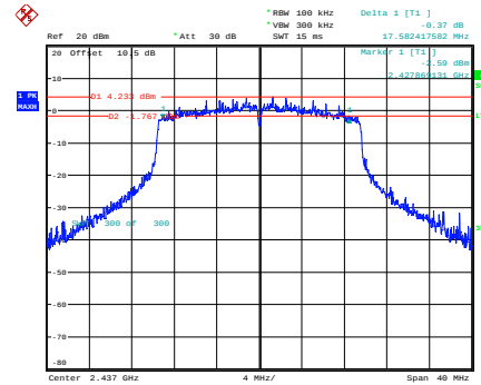
ax20_2437MHz
