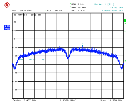
b_2437MHz
