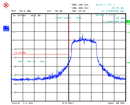
ax20_2412MHz
