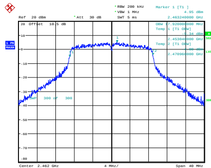
n20_2462MHz
