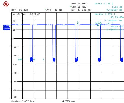
b_2437MHz
