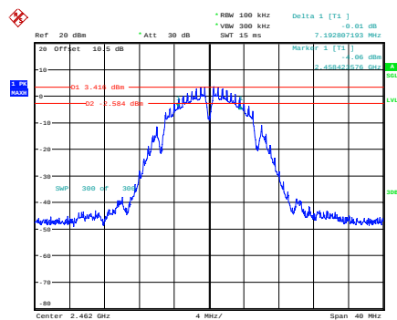
b_2462MHz
