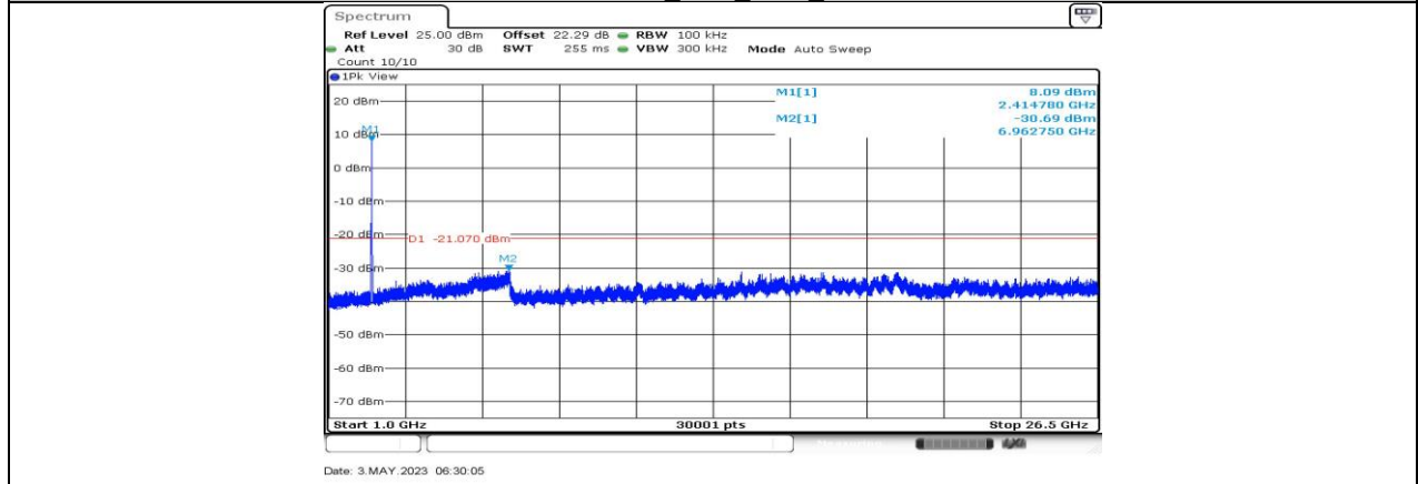
11AX20MIMO_Ant4_2417_1000-26500
