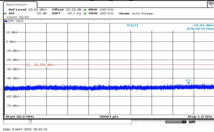
11AX40MIMO_Ant4_2422_30-1000
