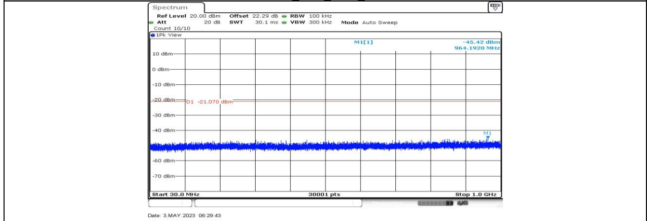
11AX20MIMO_Ant4_2417_30-1000
