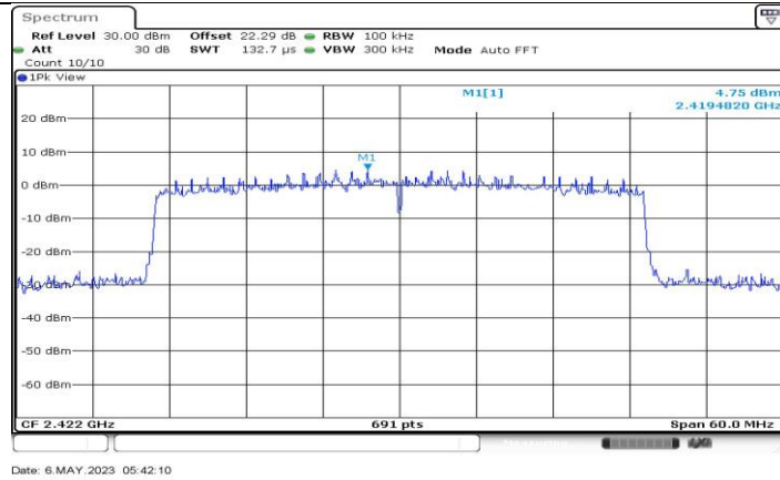
11AX40MIMO_Ant4_2422_0-Reference
