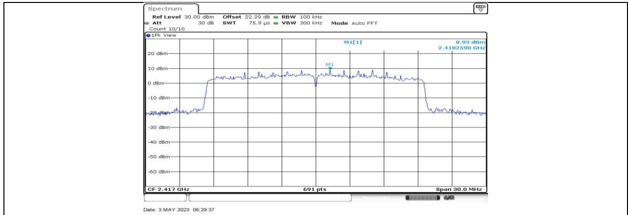
11AX20MIMO_Ant4_2417_0-Reference
