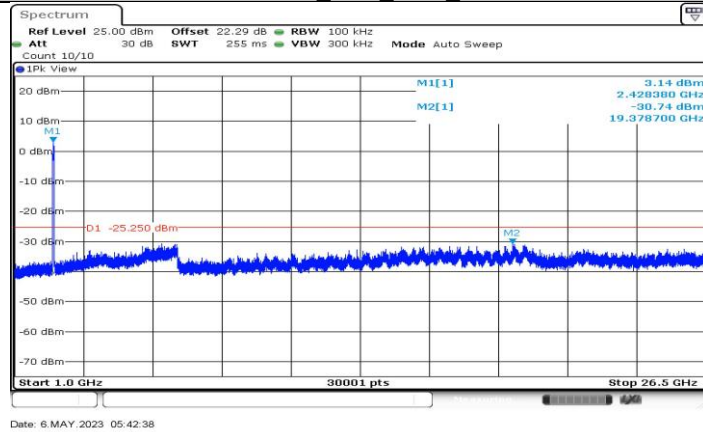
11AX40MIMO_Ant4_2422_1000-26500
