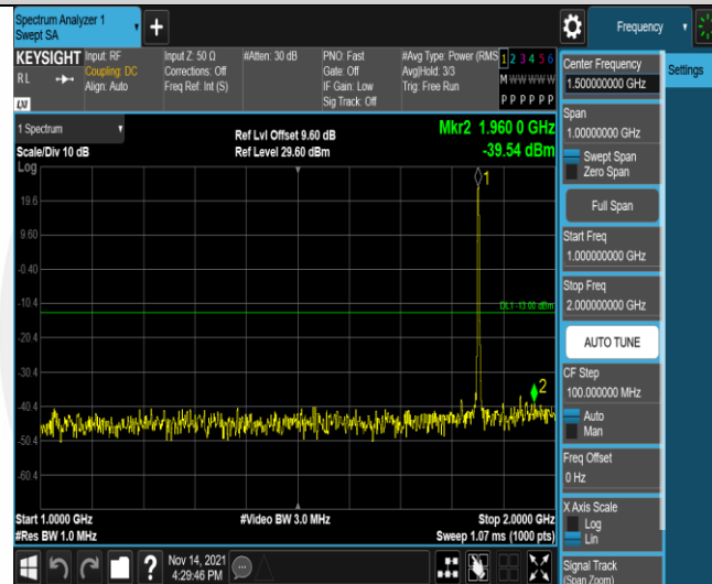
Band2-3MHz-16QAM-18615-1RB#0-Range2:1000~2000MHz
