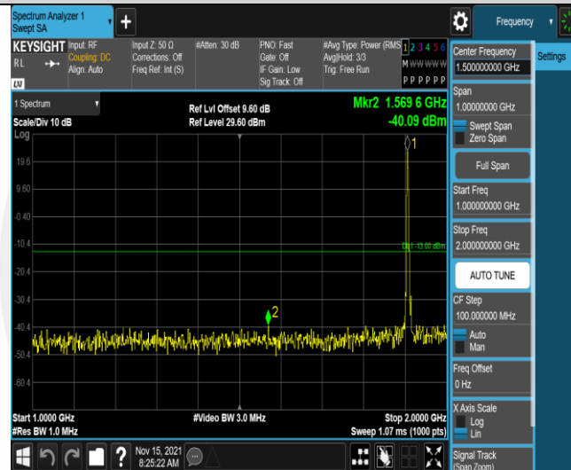
Band2-5MHz-QPSK-19175-1RB#0-Range2:1000~2000MHz
