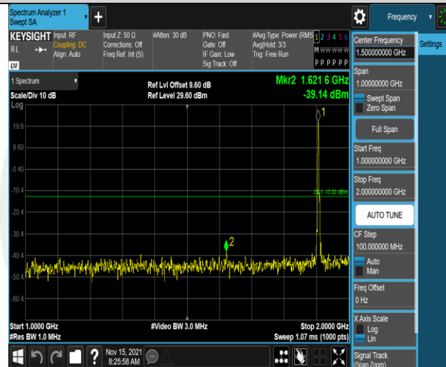
Band2-5MHz-16QAM-19175-1RB#0-Range2:1000~2000MHz
