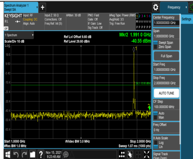
Band2-5MHz-QPSK-18900-1RB#0-Range2:1000~2000MHz
