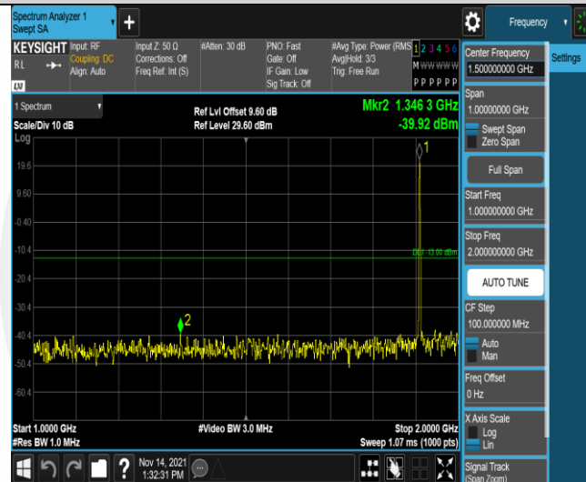
Band2-1.4MHz-QPSK-19193-1RB#0-Range2:1000~2000MHz
