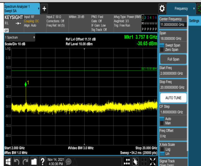
Band2-3MHz-QPSK-18900-1RB#0-Range3:2000~20000MHz
