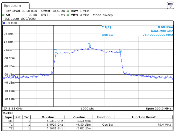
802.11ac80_5530MHz_Chain 1
