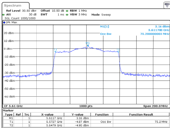
802.11ac80_5610MHz_Chain 1
