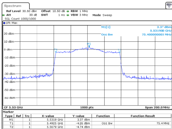
802.11ac80_5530MHz_Chain 2
