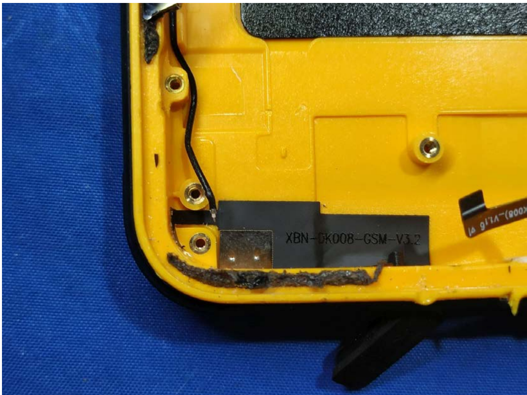
GSM ANT
