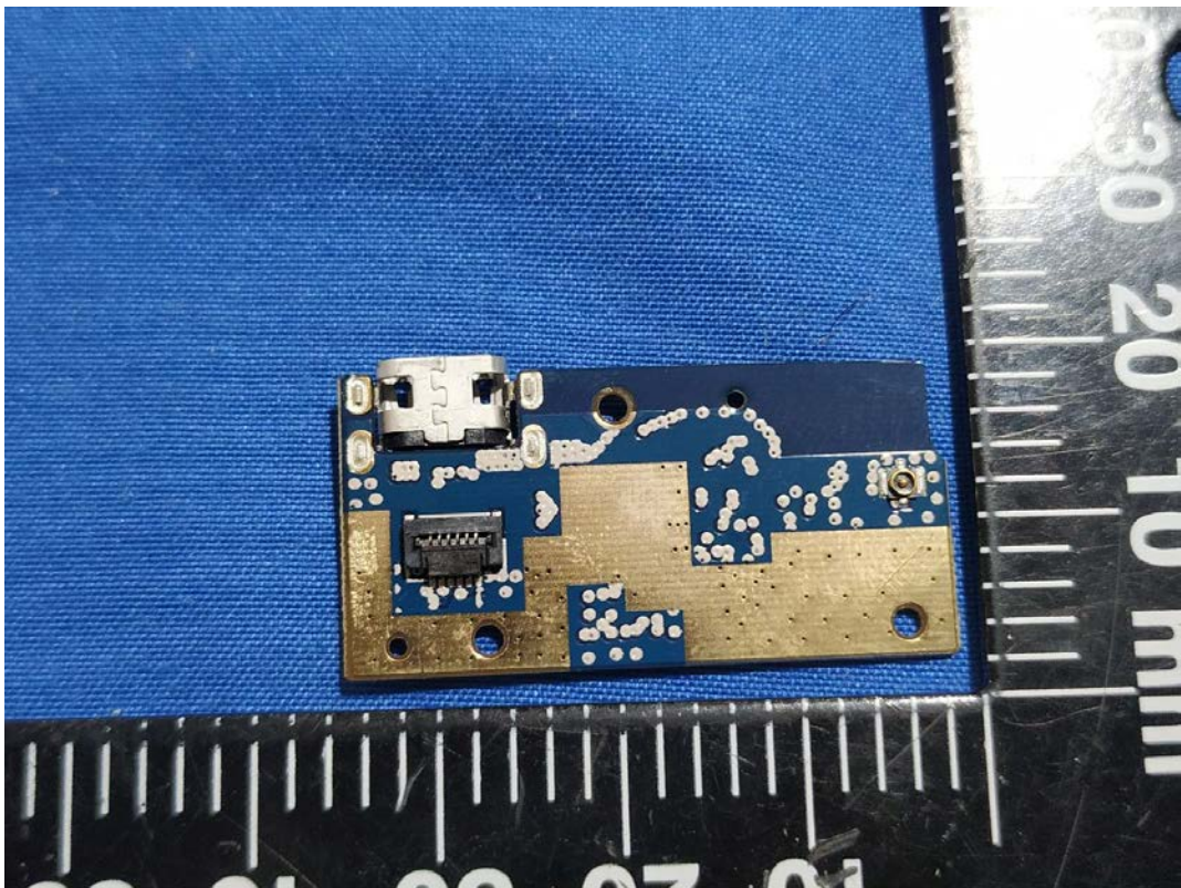
GSM ANT
