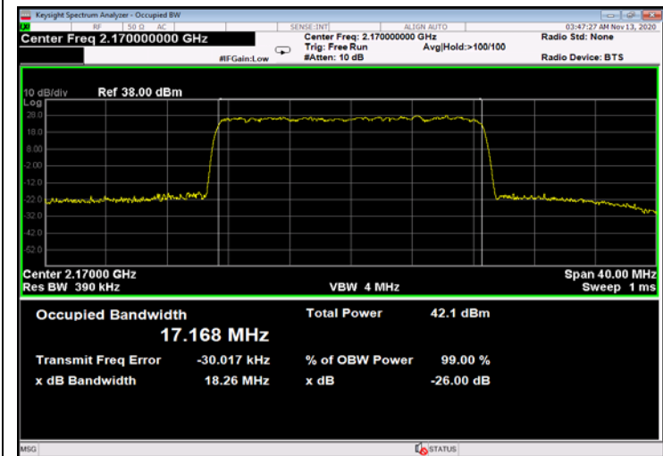
Figure 701: 256QAM 20MHz B.W.; 2170.0MHz, 60kHz - Output
