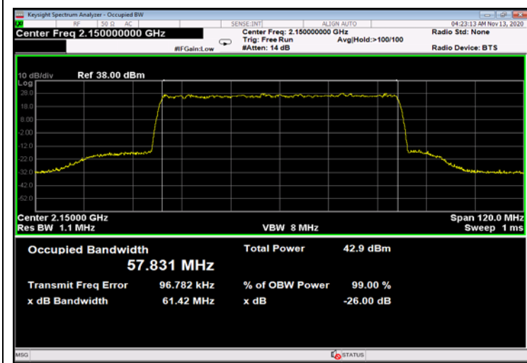
Figure 733: 256QAM 60MHz B.W.; 2150.0MHz, 30kHz - Output
