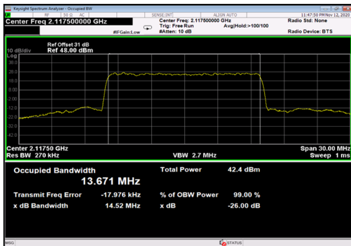
Figure 751: QPSK 15MHz B.W.; 2117.5MHz, 30kHz - Output
