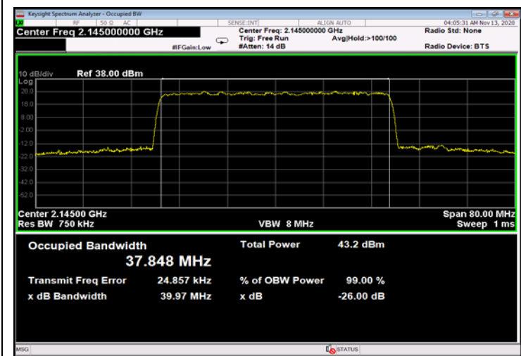
Figure 715: 256QAM 40MHz B.W.; 2145.0MHz, 30kHz - Output
