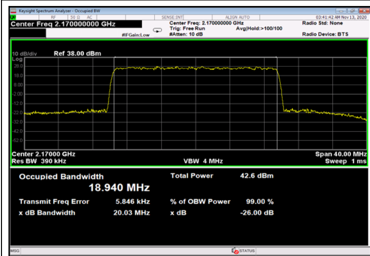
Figure 699: 256QAM 20MHz B.W.; 2170.0MHz, 15kHz - Output
