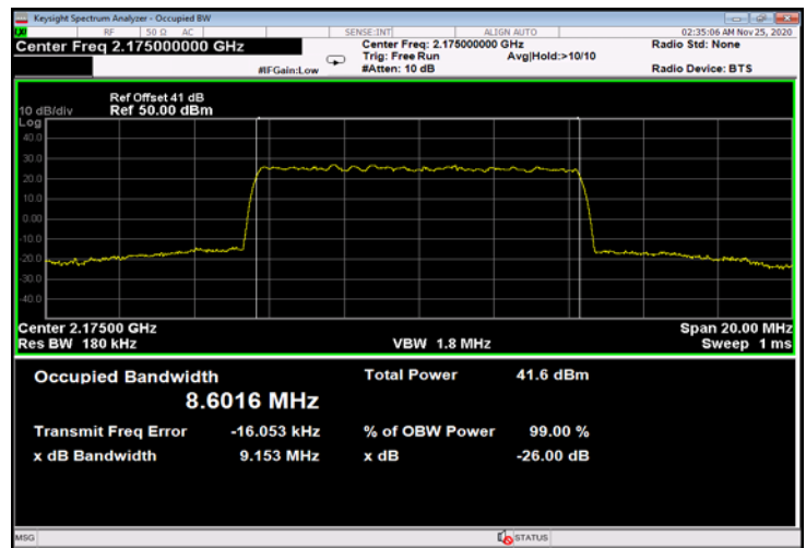
Figure 748: QPSK 10MHz B.W.; 2175.0MHz, 30kHz - Output
