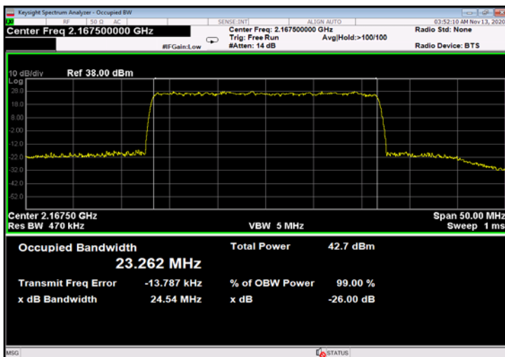
Figure 709: 256QAM 25MHz B.W.; 2167.5MHz, 30kHz - Output
