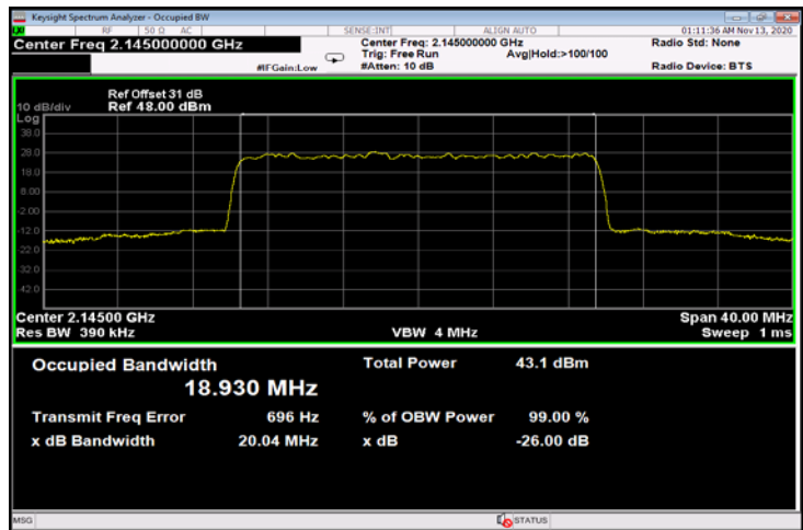
Figure 762: QPSK 20MHz B.W.; 2145.0MHz, 15kHz - Output
