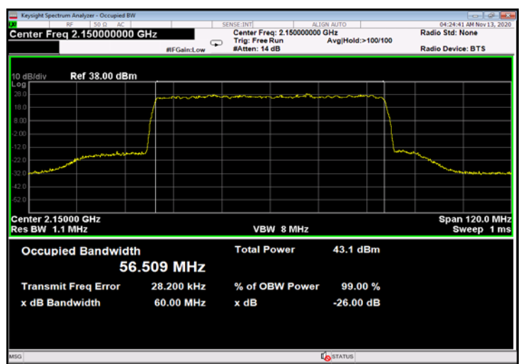
Figure 734: 256QAM 60MHz B.W.; 2150.0MHz, 60kHz - Output
