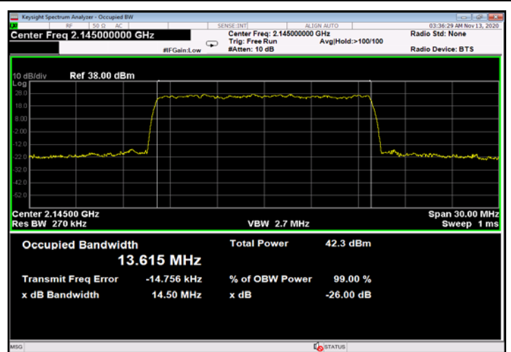
Figure 688: 256QAM 15MHz B.W.; 2145.0MHz, 30kHz - Output
