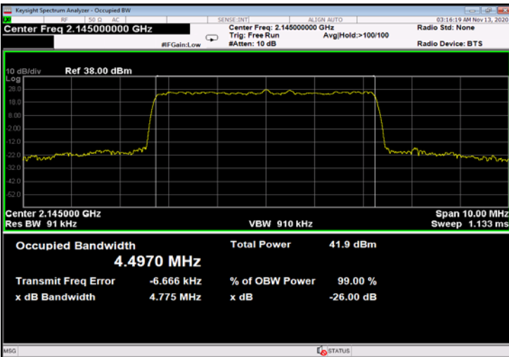
Figure 671: 256QAM 5MHz B.W.; 2145.0MHz, 15kHz - Output
