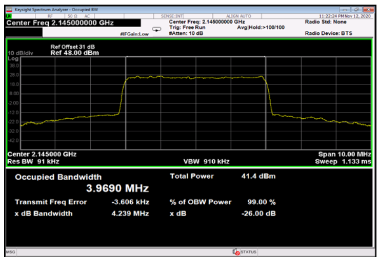
Figure 738: QPSK 5MHz B.W.; 2145.0MHz, 30kHz - Output
