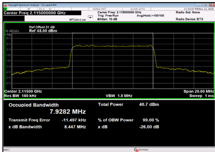
Figure 743: QPSK 10MHz B.W.; 2115.0MHz, 60kHz - Output
