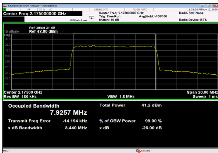
Figure 749: QPSK 10MHz B.W.; 2175.0MHz, 60kHz - Output
