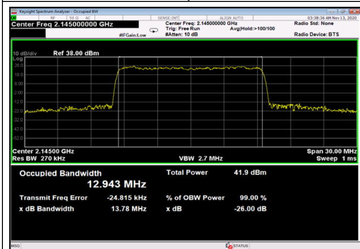
Figure 689: 256QAM 15MHz B.W.; 2145.0MHz, 60kHz - Output
