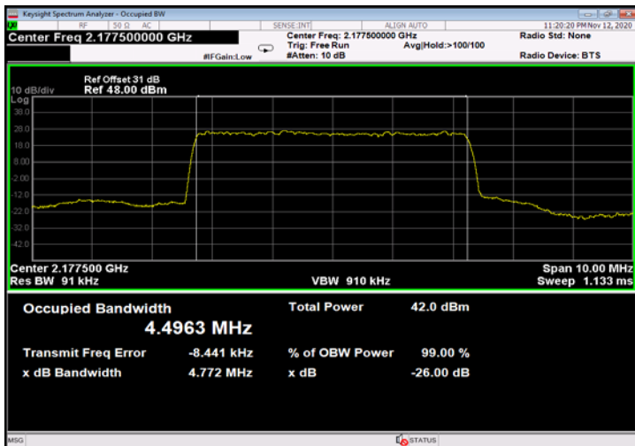
Figure 739: QPSK 5MHz B.W.; 2177.5MHz, 15kHz - Output
