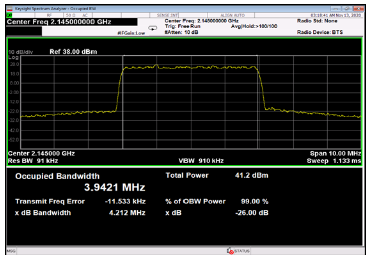
Figure 672: 256QAM 5MHz B.W.; 2145.0MHz, 30kHz - Output
