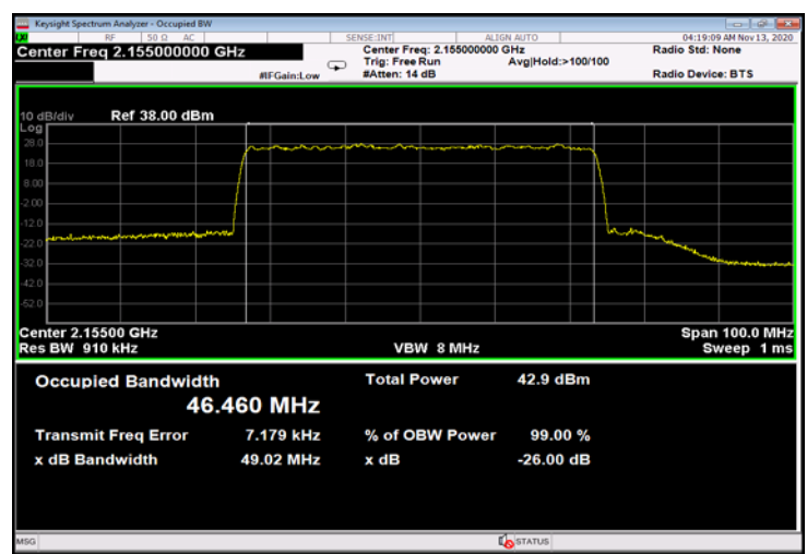
Figure 728: 256QAM 50MHz B.W.; 2155.0MHz, 60kHz - Output
