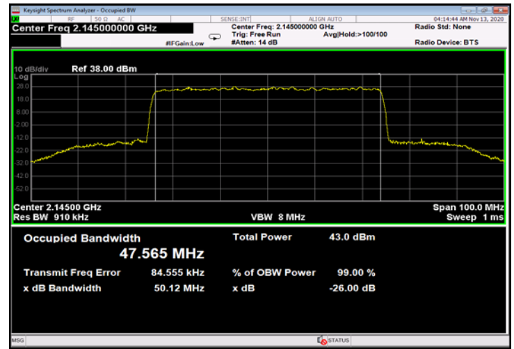
Figure 724: 256QAM 50MHz B.W.; 2145.0MHz, 30kHz - Output
