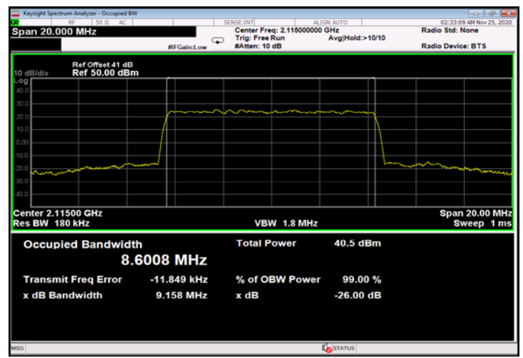
Figure 742: QPSK 10MHz B.W.; 2115.0MHz, 30kHz - Output
