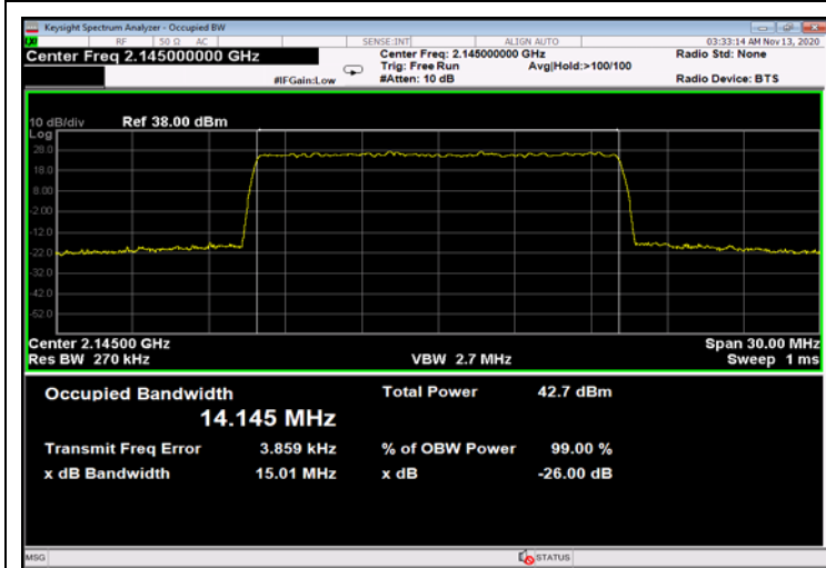
Figure 687: 256QAM 15MHz B.W.; 2145.0MHz, 15kHz - Output
