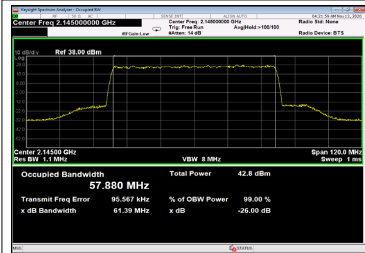
Figure 731: 256QAM 60MHz B.W.; 2145.0MHz, 30kHz - Output
