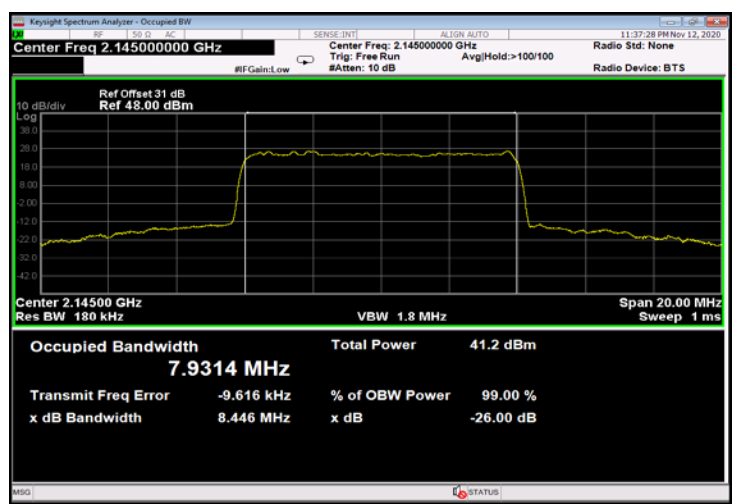
Figure 746: QPSK 10MHz B.W.; 2145.0MHz, 60kHz - Output
