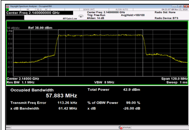
Figure 729: 256QAM 60MHz B.W.; 2140.0MHz, 30kHz - Output
