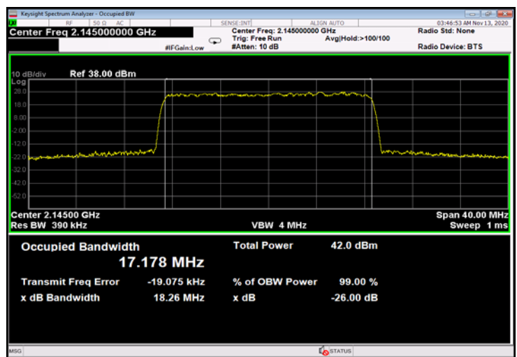
Figure 698: 256QAM 20MHz B.W.; 2145.0MHz, 60kHz - Output
