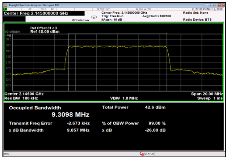
Figure 744: QPSK 10MHz B.W.; 2145.0MHz, 15kHz - Output
