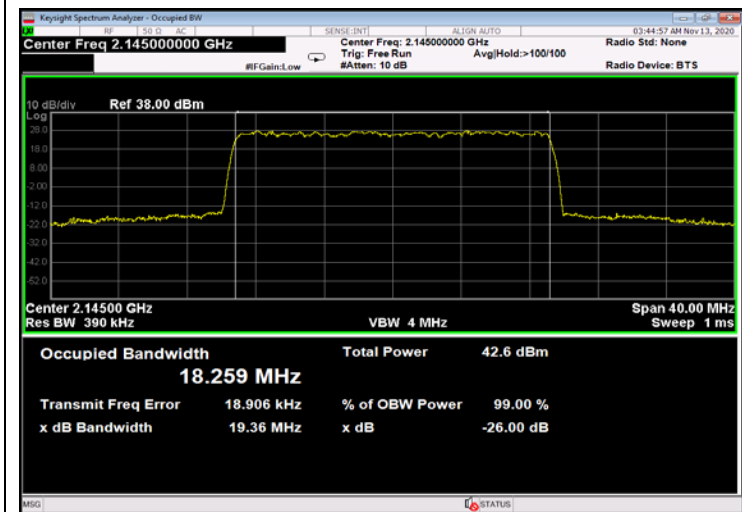
Figure 697: 256QAM 20MHz B.W.; 2145.0MHz, 30kHz - Output
