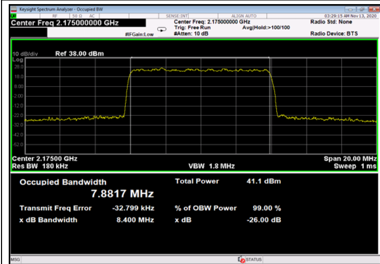
Figure 683: 256QAM 10MHz B.W.; 2175.0MHz, 60kHz - Output
