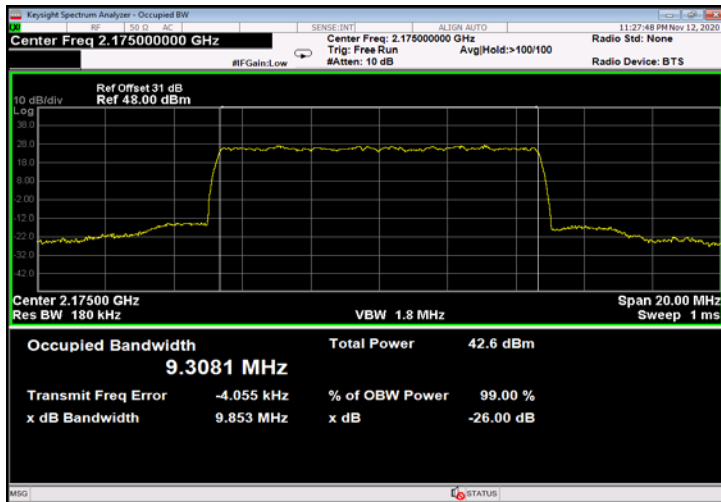
Figure 747: QPSK 10MHz B.W.; 2175.0MHz, 15kHz - Output
