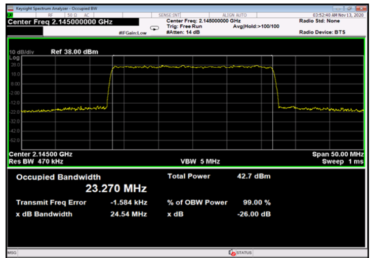
Figure 706: 256QAM 25MHz B.W.; 2145.0MHz, 30kHz - Output
