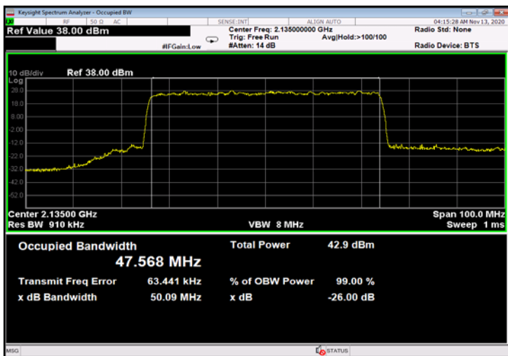
Figure 721: 256QAM 50MHz B.W.; 2135.0MHz, 30kHz - Output
