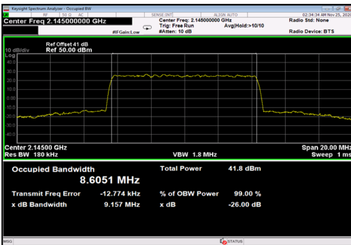
Figure 745: QPSK 10MHz B.W.; 2145.0MHz, 30kHz - Output
