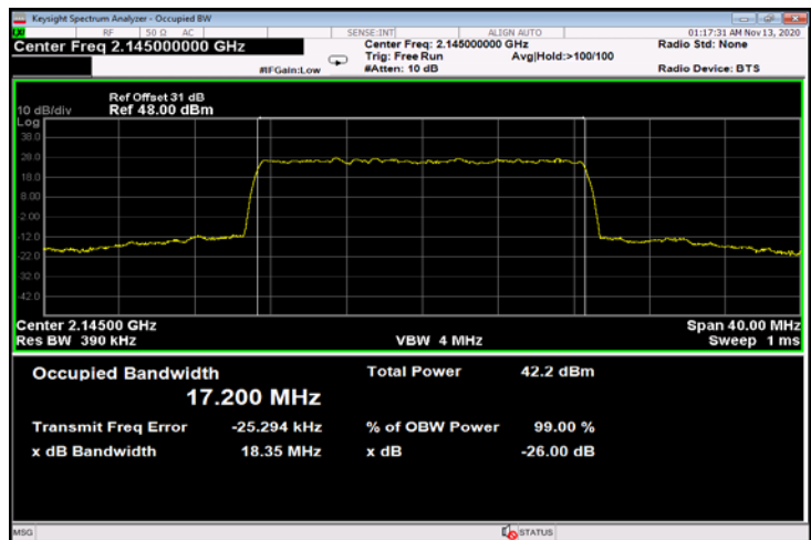
Figure 764: QPSK 20MHz B.W.; 2145.0MHz, 60kHz - Output
