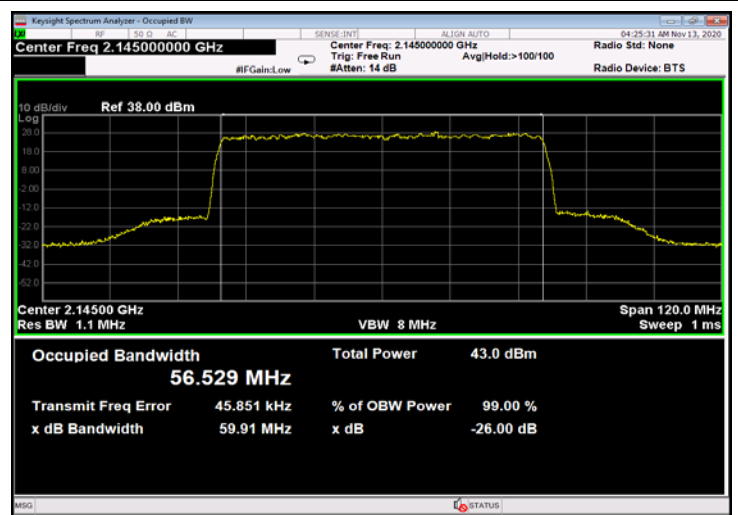
Figure 732: 256QAM 60MHz B.W.; 2145.0MHz, 60kHz - Output
