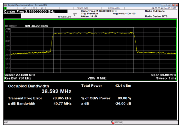
Figure 714: 256QAM 40MHz B.W.; 2145.0MHz, 15kHz - Output
