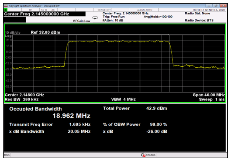
Figure 696: 256QAM 20MHz B.W.; 2145.0MHz, 15kHz - Output
