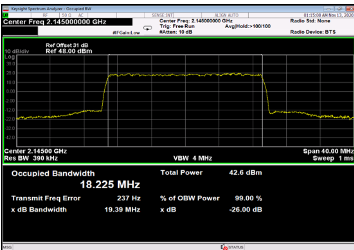
Figure 763: QPSK 20MHz B.W.; 2145.0MHz, 30kHz - Output
