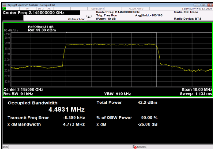
Figure 737: QPSK 5MHz B.W.; 2145.0MHz, 15kHz - Output
