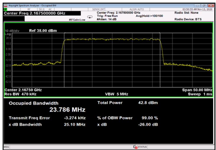
Figure 708: 256QAM 25MHz B.W.; 2167.5MHz, 15kHz - Output
