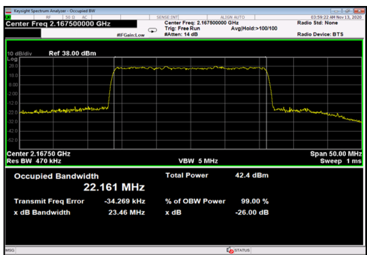
Figure 710: 256QAM 25MHz B.W.; 2167.5MHz, 60kHz - Output
