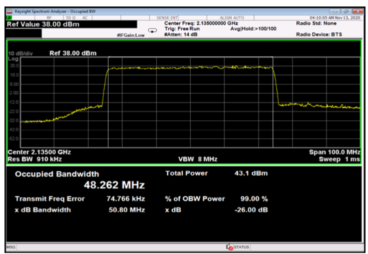
Figure 720: 256QAM 50MHz B.W.; 2135.0MHz, 15kHz - Output
