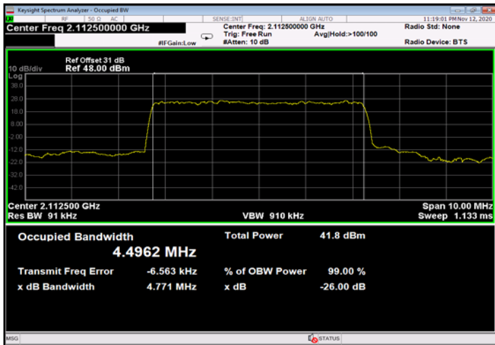
Figure 735: QPSK 5MHz B.W.; 2112.5MHz, 15kHz - Output
