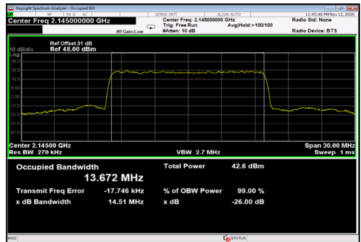
Figure 754: QPSK 15MHz B.W.; 2145.0MHz, 30kHz - Output
