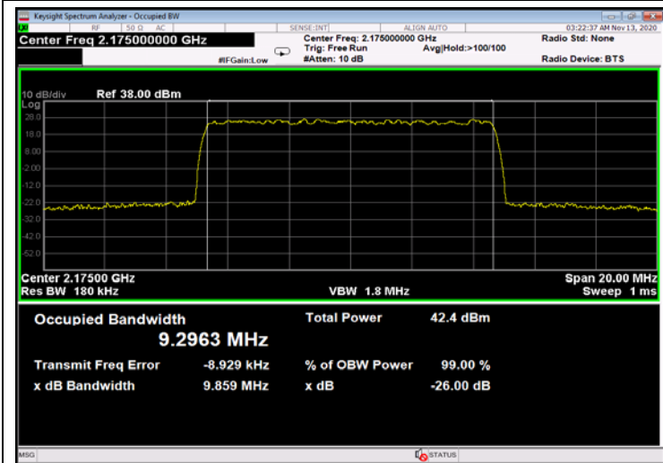
Figure 681: 256QAM 10MHz B.W.; 2175.0MHz, 15kHz - Output
