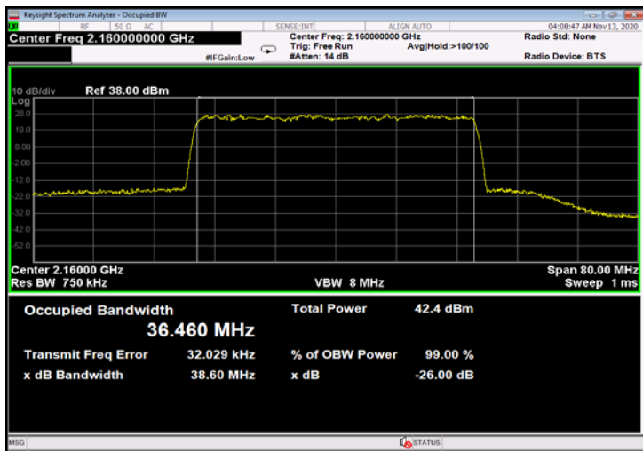
Figure 719: 256QAM 40MHz B.W.; 2160.0MHz, 60kHz - Output
