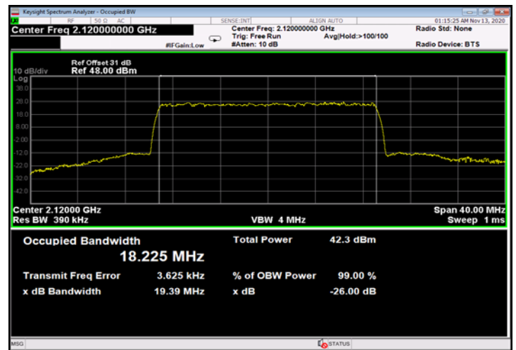
Figure 760: QPSK 20MHz B.W.; 2120.0MHz, 30kHz - Output
