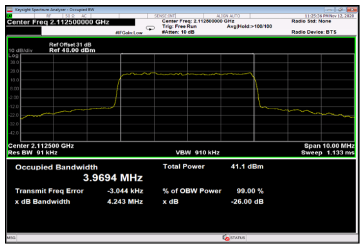
Figure 736: QPSK 5MHz B.W.; 2112.5MHz, 30kHz - Output
