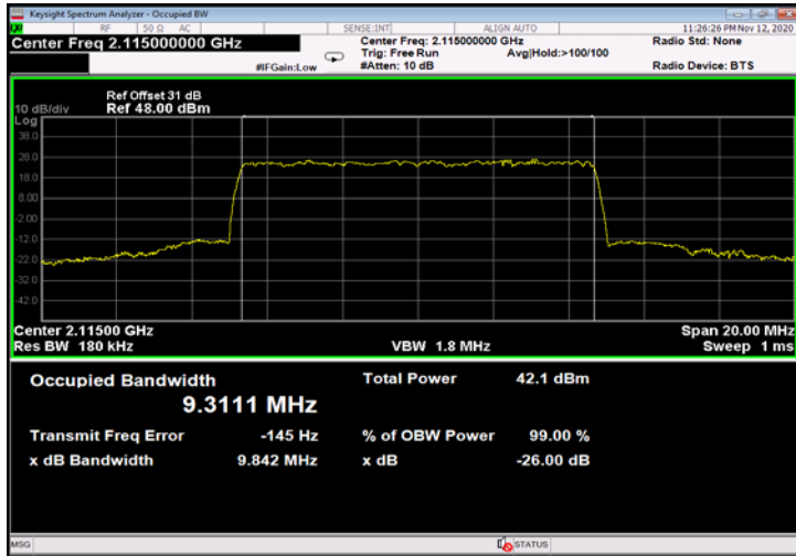
Figure 741: QPSK 10MHz B.W.; 2115.0MHz, 15kHz - Output
