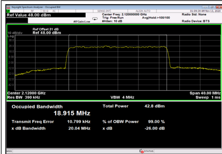
Figure 759: QPSK 20MHz B.W.; 2120.0MHz, 15kHz - Output
