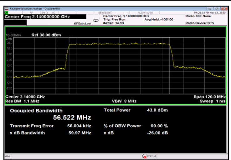
Figure 730: 256QAM 60MHz B.W.; 2140.0MHz, 60kHz - Output
