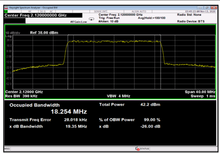
Figure 694: 256QAM 20MHz B.W.; 2120.0MHz, 30kHz - Output
