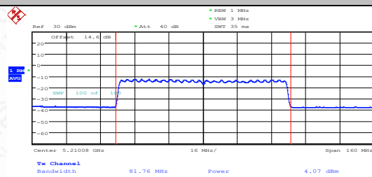
11AX80SISO-Ant1-5210-PASS
