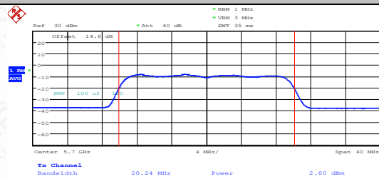
11AX20MIMO-Ant1-5700-PASS
