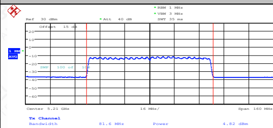
11AX80SISO-Ant2-5210-PASS
