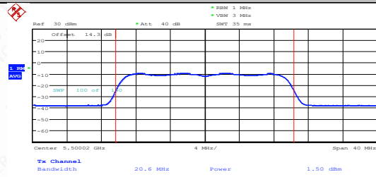
11AX20MIMO-Ant1-5500-PASS
