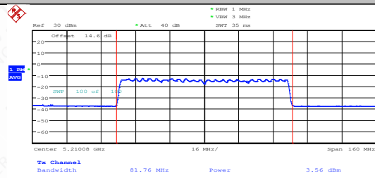
11AX80MIMO-Ant1-5210-PASS
