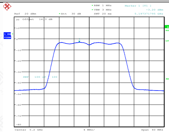
11N20MIMO-Ant1-5200-PASS
