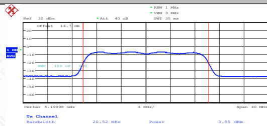
11AX20MIMO-Ant1-5200-PASS
