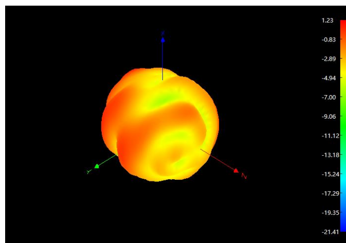
2500MHz 3D
