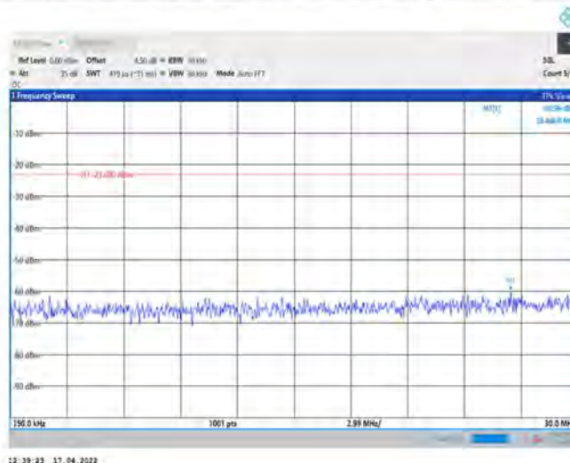
Band12-10MHz-QPSK-23060-1RB#0-Range2:0.15~30MHz
