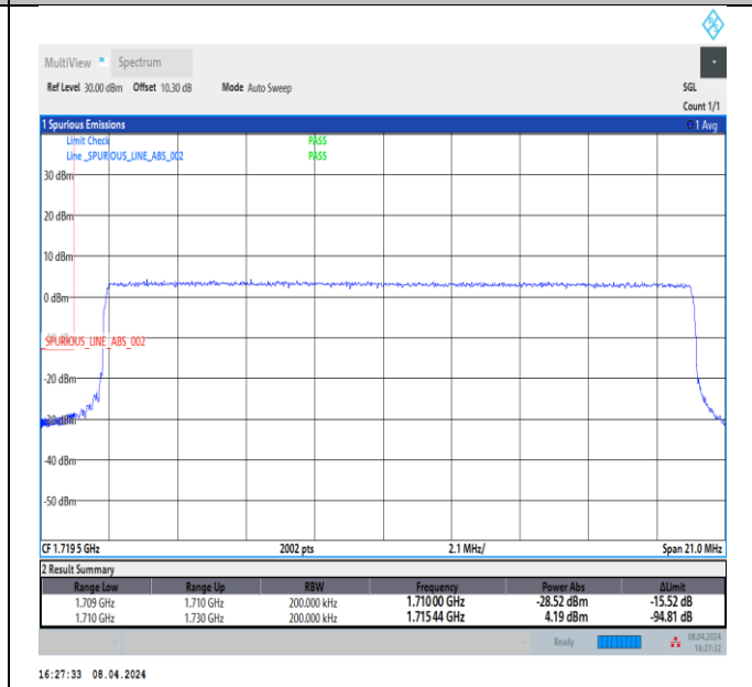
Band66_20MHz_QPSK_132072_100RB#0
