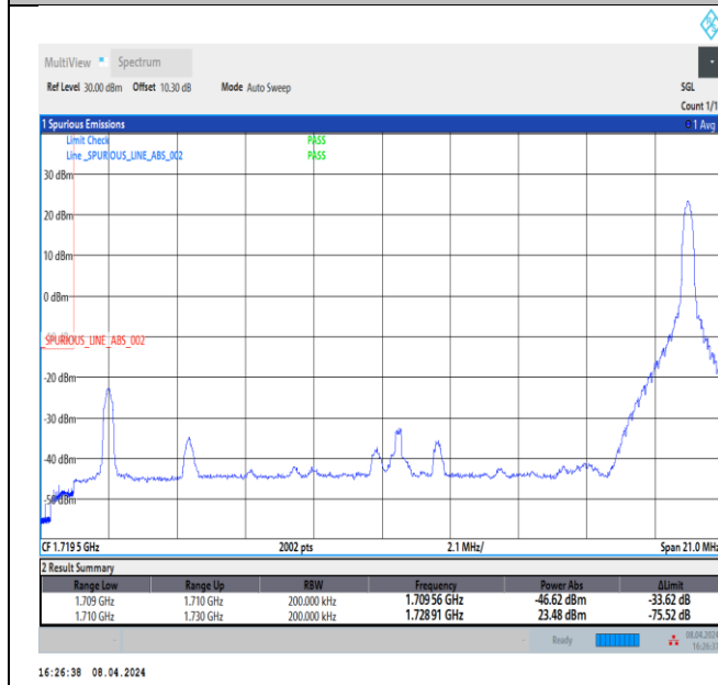
Band66_20MHz_QPSK_132072_1RB#99
