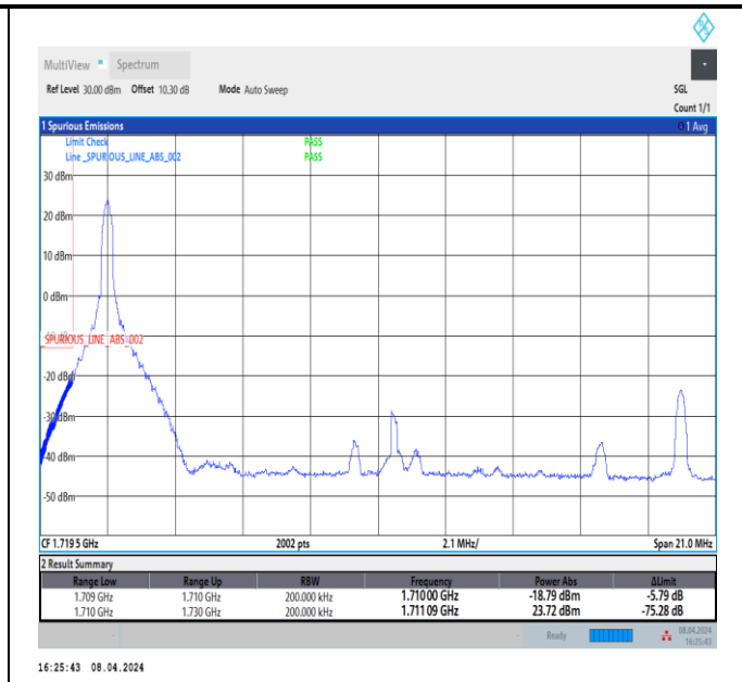
Band66_20MHz_QPSK_132072_1RB#0
