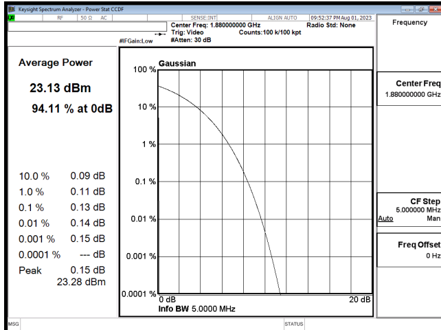
PTAR 2G1900 CH661 EGPRS
