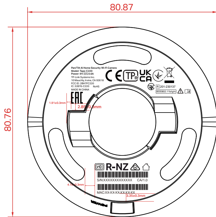
尺寸图
