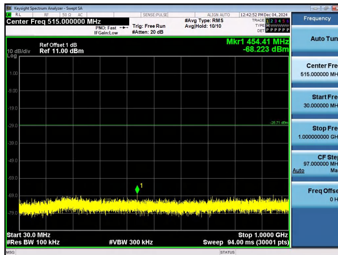
11G-Ant1-2437-30~1000-PASS
