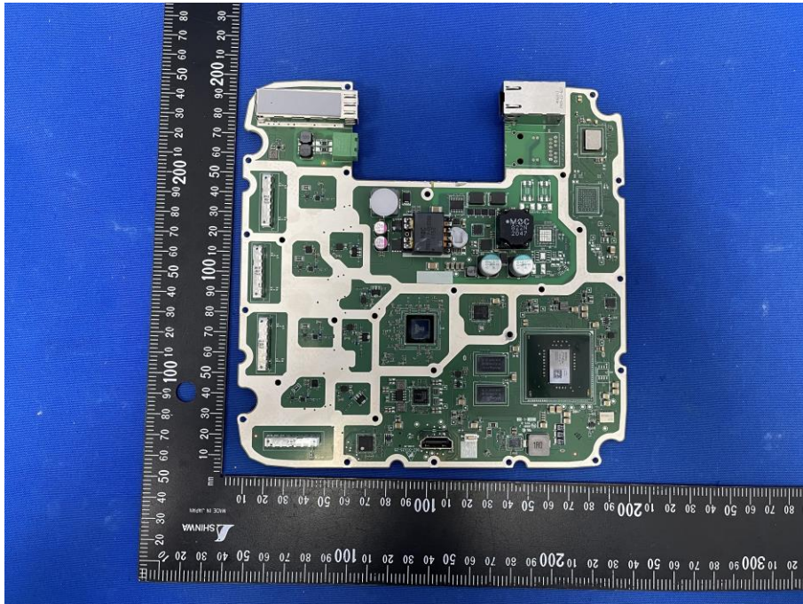
(9) EUT Photo
