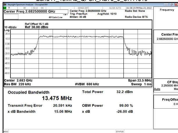
Band41_15MHz_QPSK_RB75_0_CH41515
