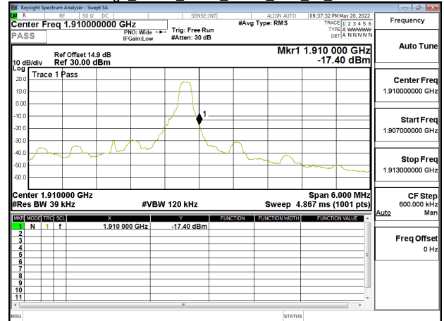
Band Edge_Band2_3MHz_QPSK_RB1_14_CH19185
