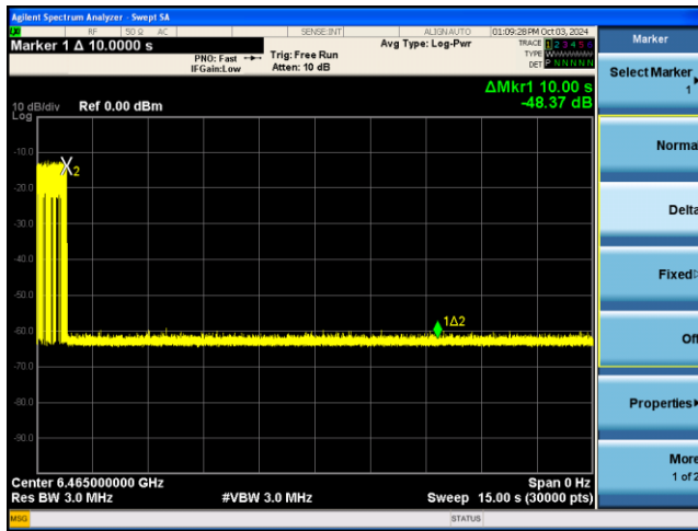
BE80-6465MHz-Inc1
