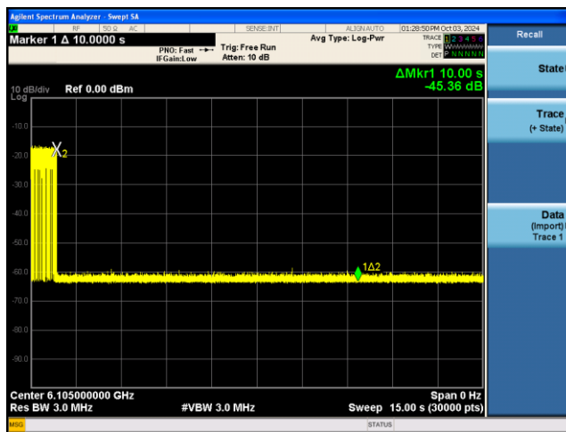
BE320-6105MHz -Inc3
