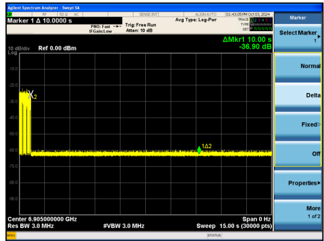
BE320-6905MHz -Inc2
