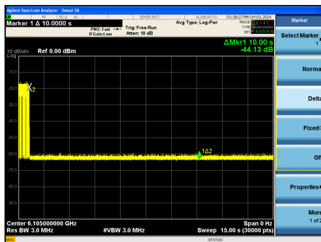
BE320-6105MHz -Inc2
