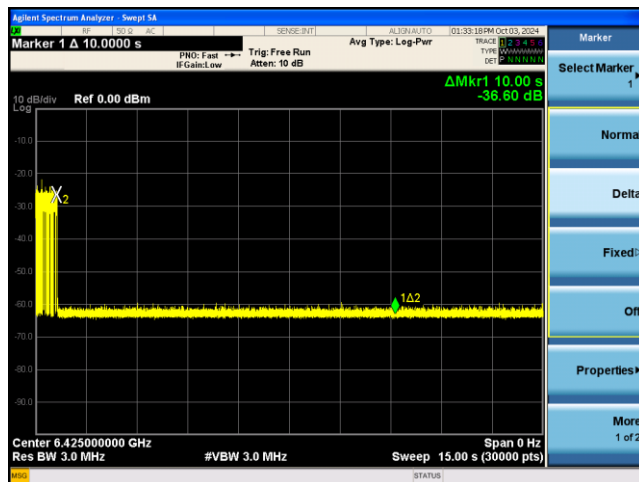
BE320-6425MHz -Inc2
