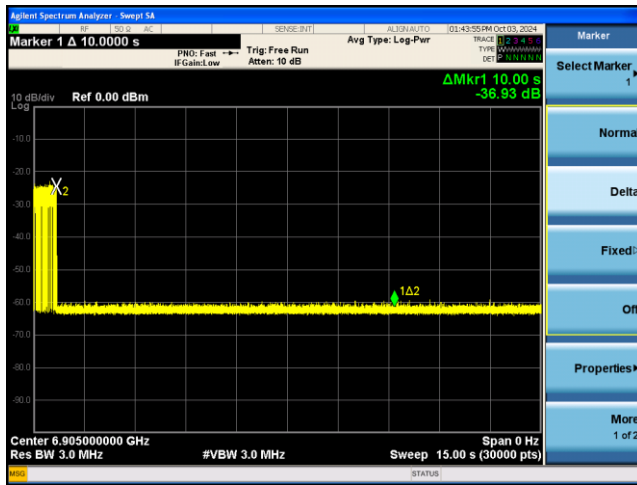
BE320-6905MHz-Inc1
