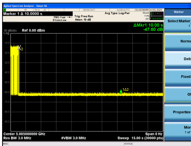
BE80-5985MHz-Inc3
