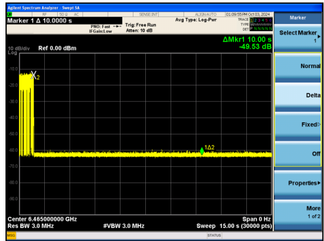
BE80-6465MHz -Inc2
