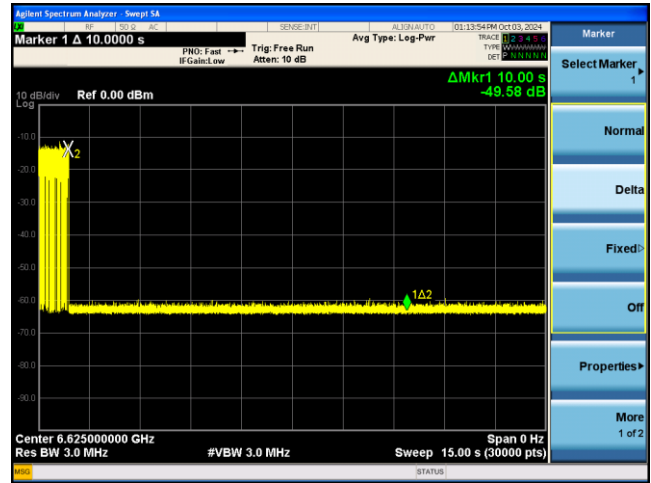
BE80-6625MHz -Inc2
