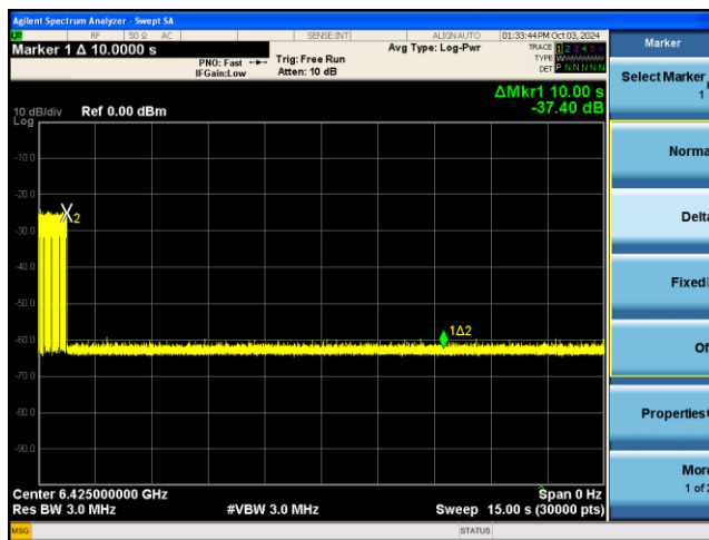
BE320-6425MHz -Inc3
