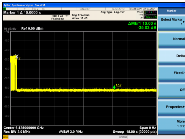
BE320-6425MHz-Inc1
