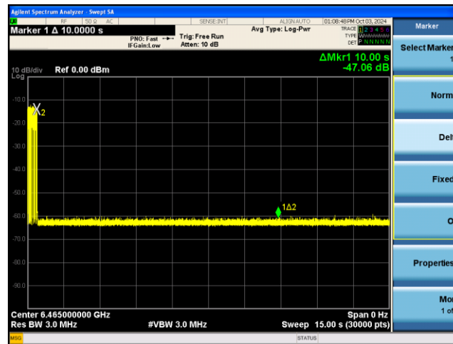
BE80-6465MHz -Inc3
