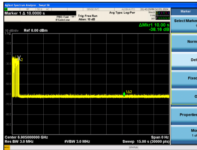
BE320-6905MHz -Inc3
