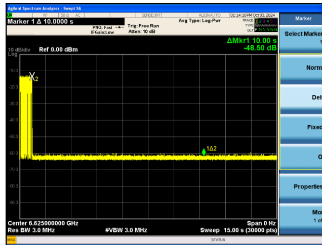
BE80-6625MHz -Inc3
