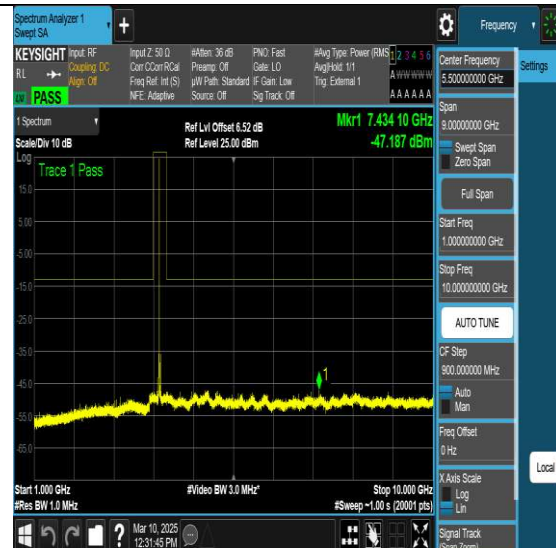
NTNV-N77-3700-3980-PC2-30-40-M-DFT-QPSK- Edge 1RB Left-Ant1-PASS
