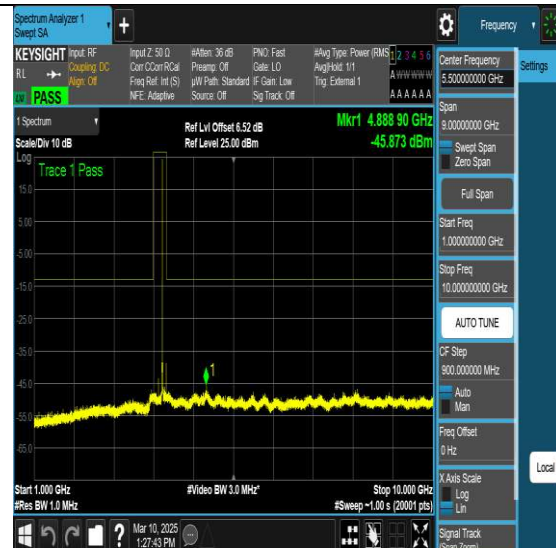
NTNV-N77-3700-3980-PC2-30-90-H-DFT-QPSK- Edge 1RB Left-Ant1-PASS
