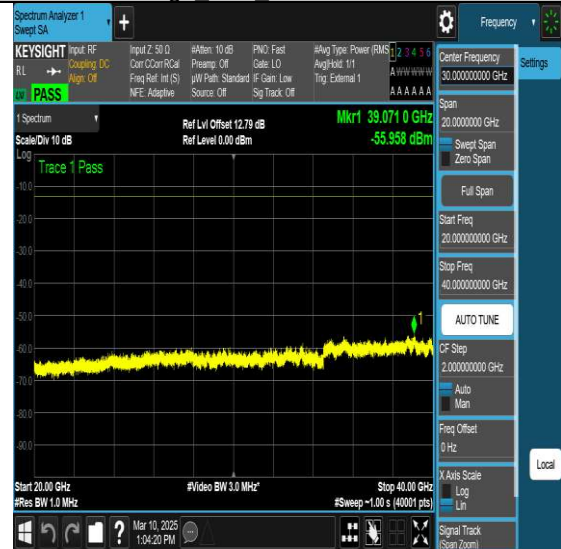
NTNV-N77-3700-3980-PC2-30-70-M-DFT-QPSK- Edge 1RB Left-Ant1-PASS
