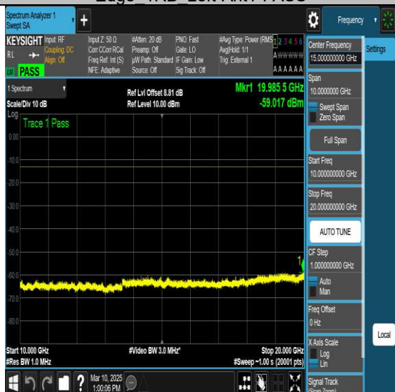
NTNV-N77-3700-3980-PC2-30-70-L-DFT-QPSK- Edge 1RB Left-Ant1-PASS
