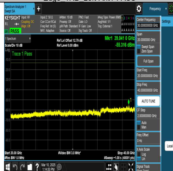
NTNV-N77-3700-3980-PC2-30-80-M-DFT-QPSK- Edge 1RB Left-Ant1-PASS
