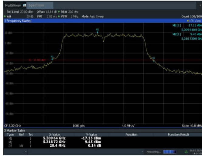
11A_ANT10_5320
