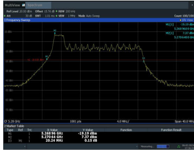
11AX20MIMO_ANT7_5280_52Tone_RU37
