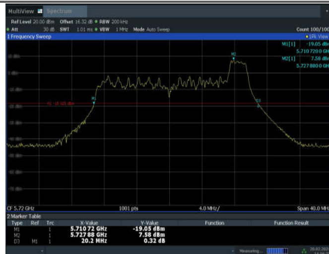
11AX20MIMO_ANT10_5720_26Tone_RU8
