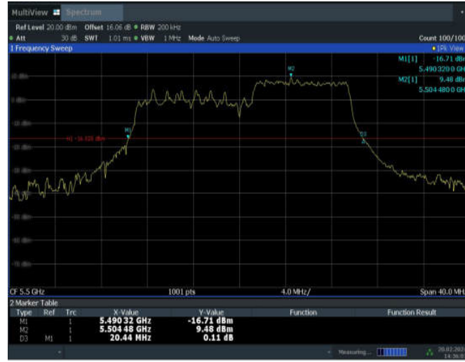
11AX20MIMO_ANT10_5500_106Tone_RU54
