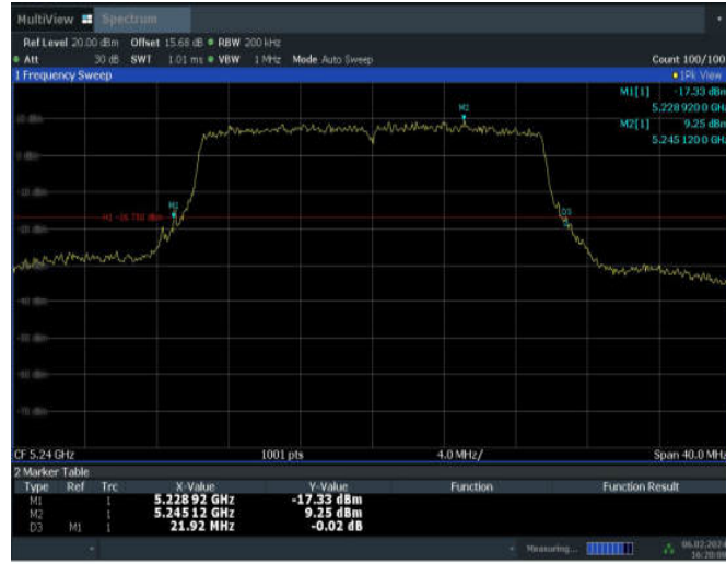
11AX20MIMO_ANT10_5240
