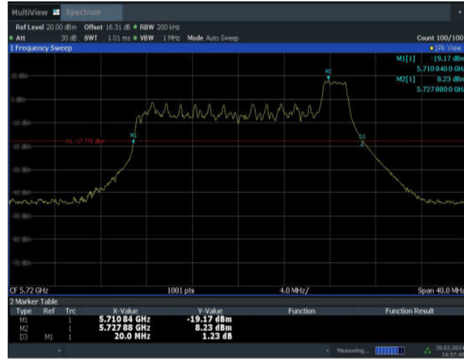
11AX20MIMO_ANT7_5720_52Tone_RU40
