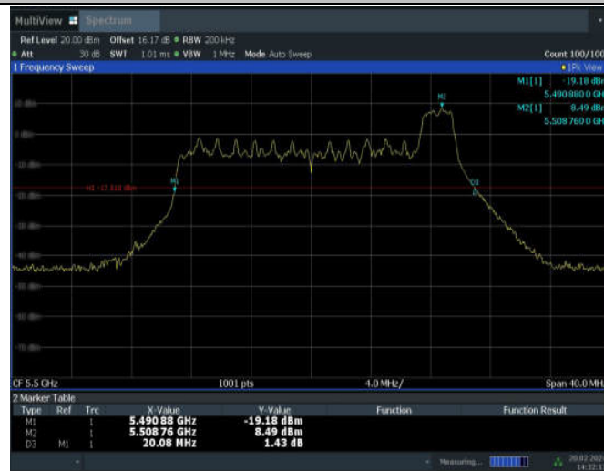
11AX20MIMO_ANT7_5500_26Tone_RU8
