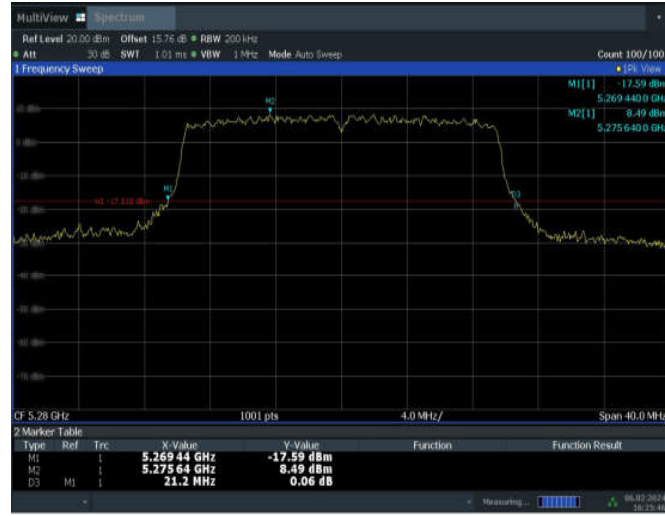
11AX20MIMO_ANT7_5280
