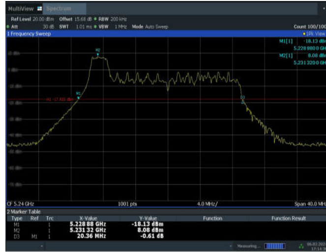
11AX20MIMO_ANT10_5240_52Tone_RU37
