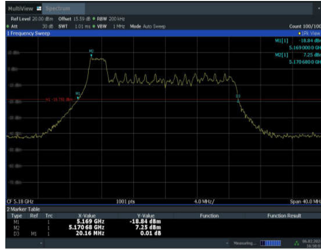
11AX20MIMO_ANT7_5180_26Tone_RU0
