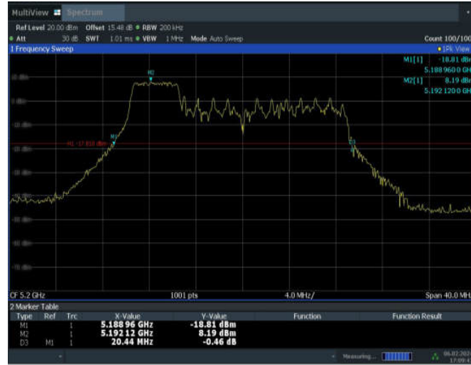
11AX20MIMO_ANT10_5200_106Tone_RU53
