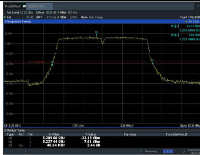
11AC40SISO_ANT10_5230
