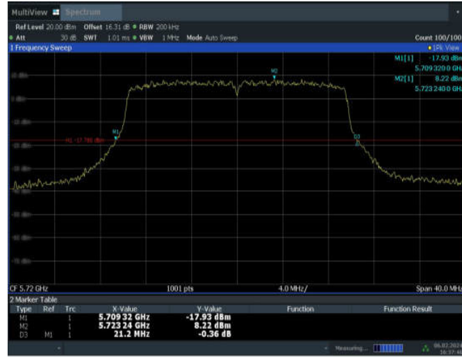
11AX20MIMO_ANT7_5720
