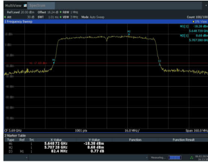
11AC80MIMO_ANT7_5690
