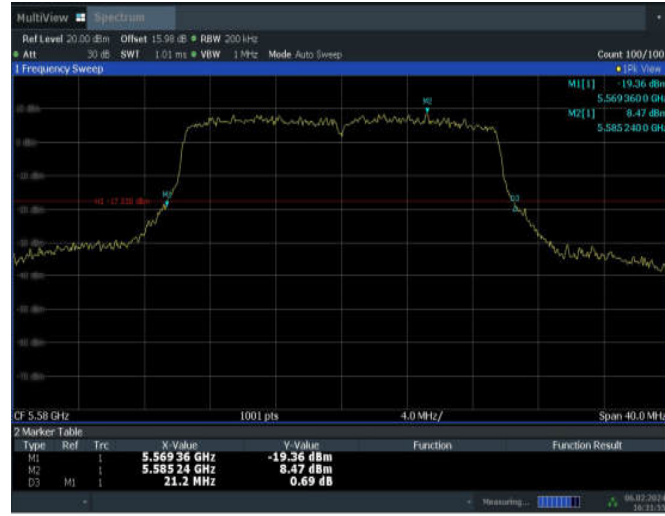
11AX20MIMO_ANT10_5580
