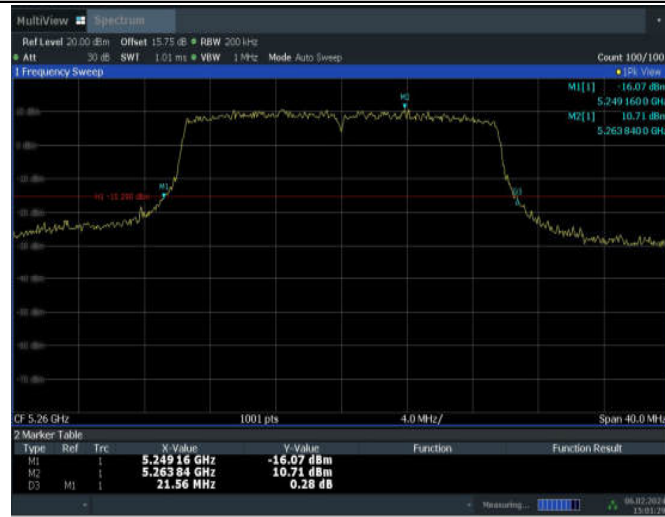
11AX20SISO_ANT10_5260
