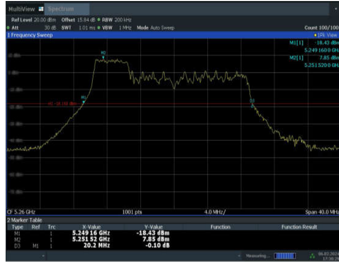
11AX20MIMO_ANT7_5260_106Tone_RU53
