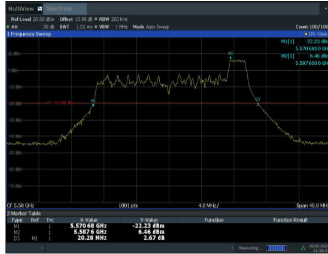
11AX20MIMO_ANT10_5580_52Tone_RU40
