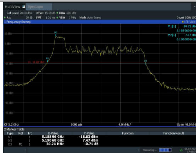
11AX20MIMO_ANT7_5200_26Tone_RU0
