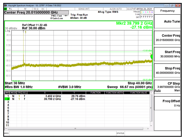
5G NR n77 60MHz QPSK Low Channel RB1-1
