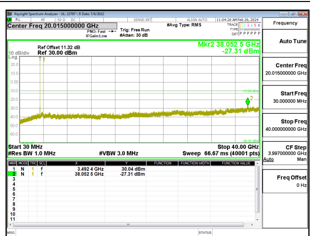
5G NR n77 20MHz QPSK Mid Channel RB1-0
