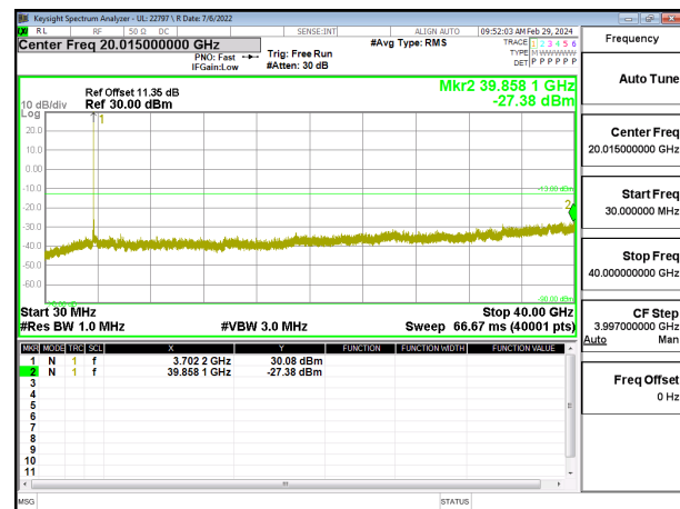
5G NR n77 60MHz QPSK Mid Channel RB1-1
