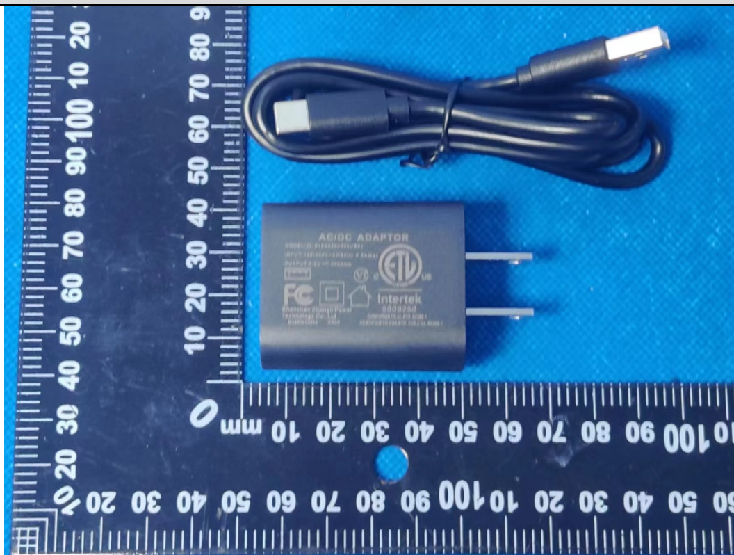
EUT Photo
