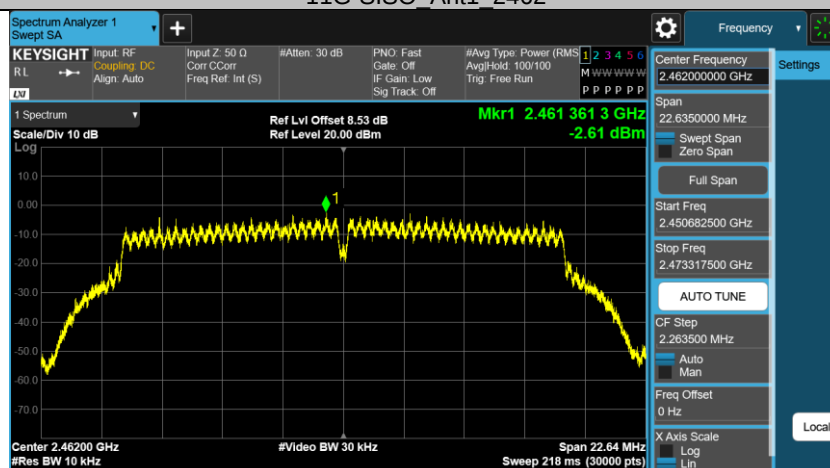
11G-SISO_Ant1_2462
