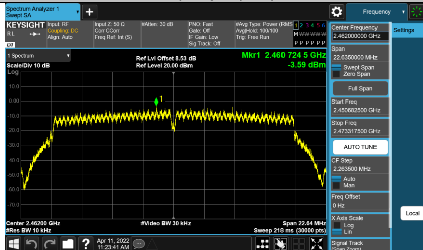
11N20MIMO Ant2 2462
