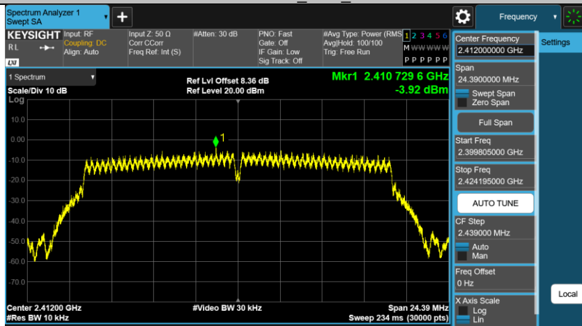
11N20MIMO_Ant2_2412
