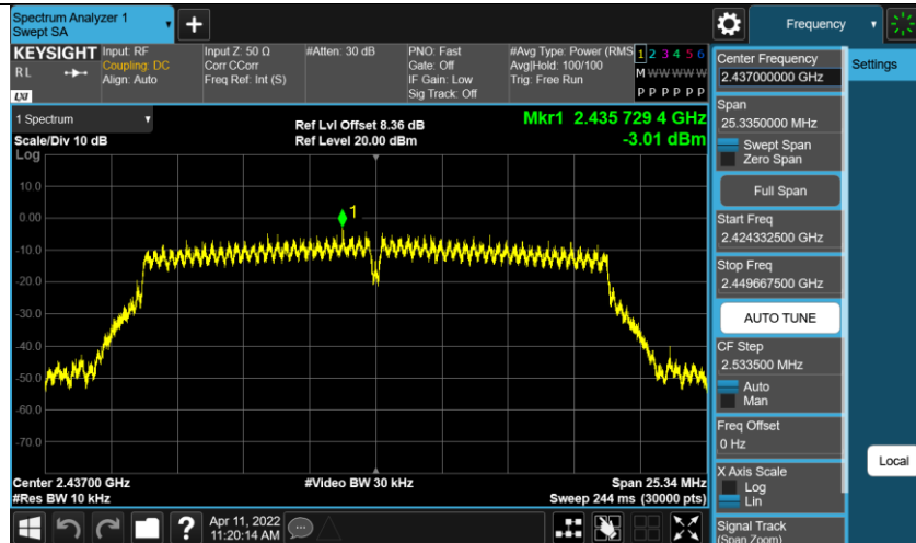
11N20MIMO Ant2 2437
