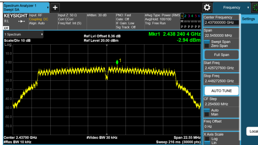
11G-SISO_Ant2_2437
