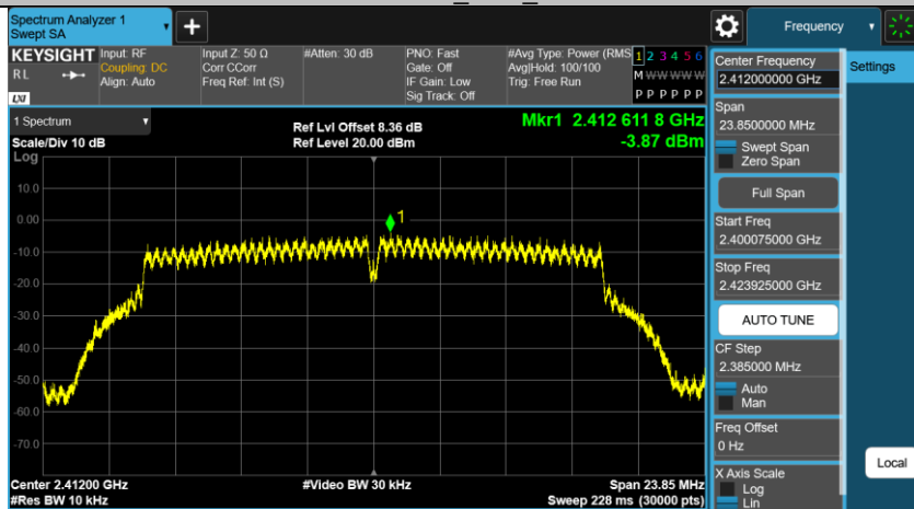
11G-SISO_Ant2_2412
