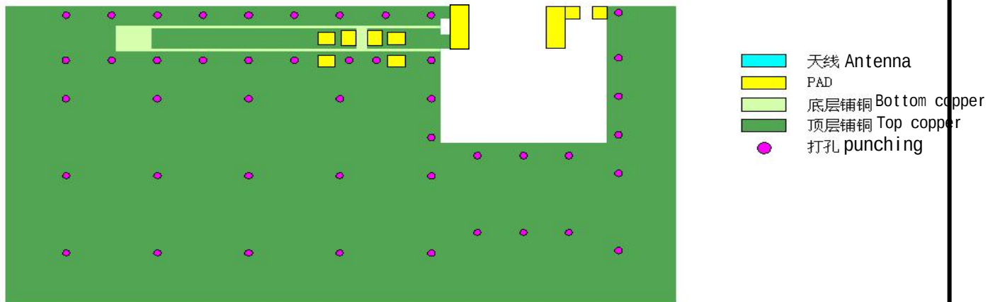
打孔参考示意图 Punching reference diagram
