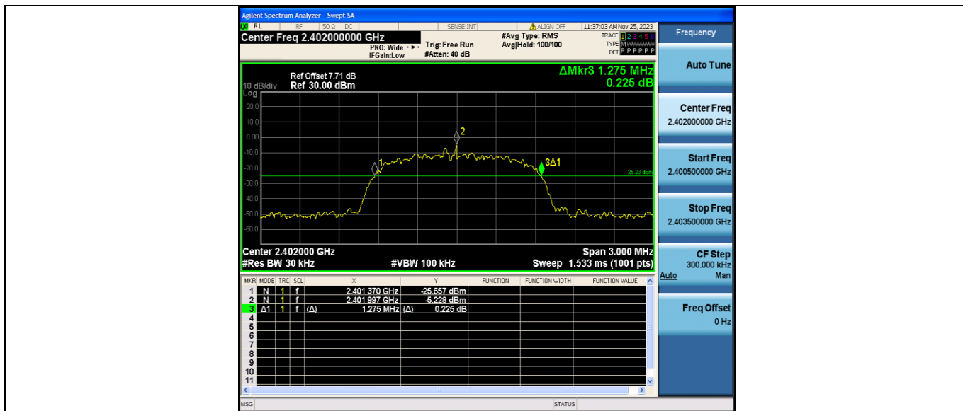
3DH5_Ant2_2402
