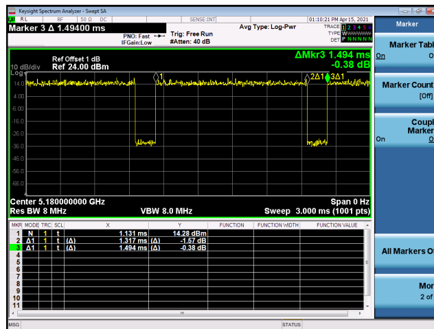
IEEE 802.11ac(VHT20)
