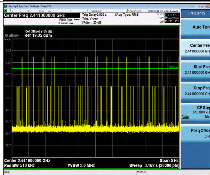
DH3_Ant0_Hop
