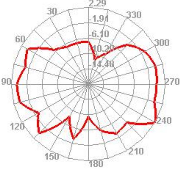
2450.000MHz E2
