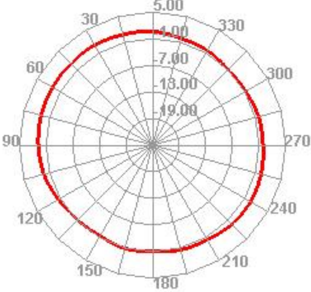
2450.000MHz H
