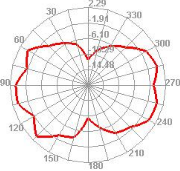
2450.000MHz E1
