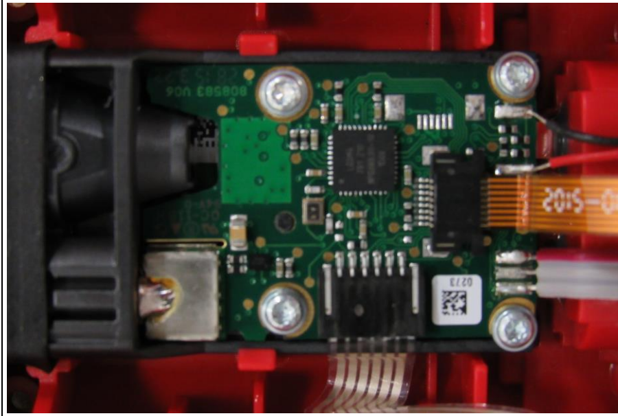
EUT PCB
