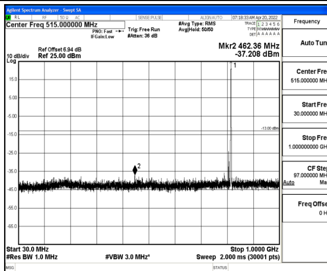
Band26-1.4MHz-16QAM-26740-1-0-Low-30-1000--37.21-PASS
