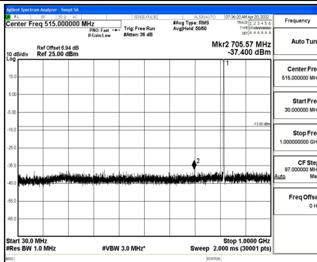
Band26-3MHz-QPSK-26740-1-0-Low-30-1000--37.4-PASS
