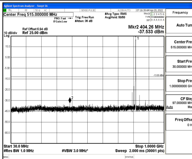
Band26-1.4MHz-QPSK-26740-1-0-Low-30-1000--37.53-PASS
