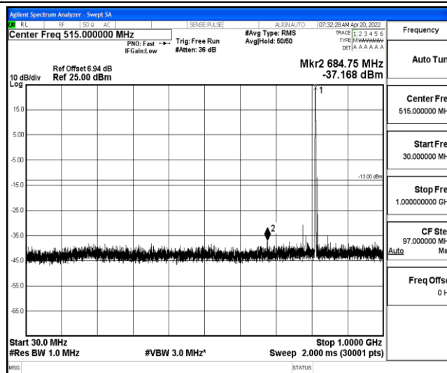
Band26-3MHz-QPSK-26705-1-0-Low-30-1000--37.17-PASS
