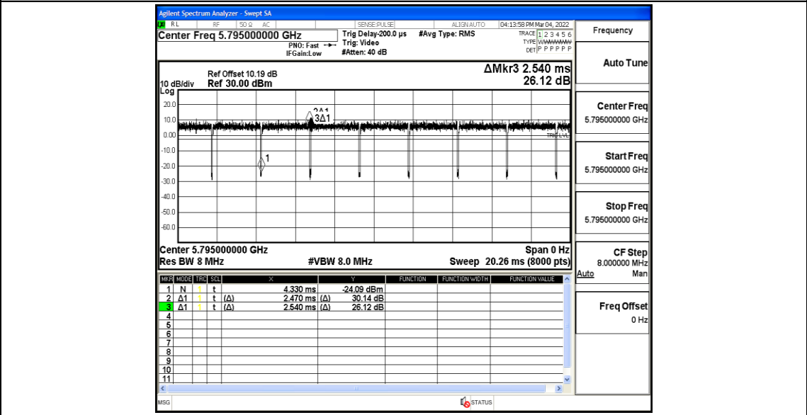
11N40MIMO_Ant1_5795
