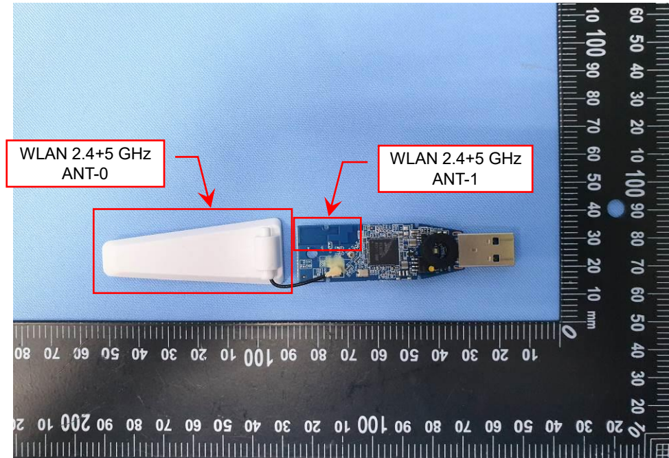
EUT Photo (4)
