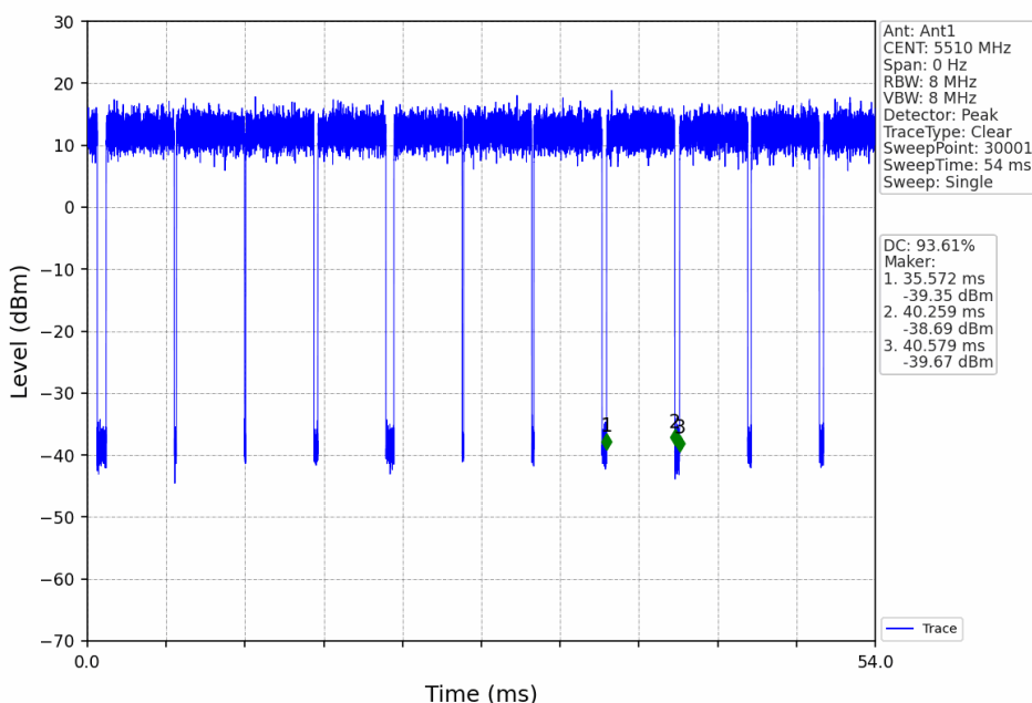
802.11be(EHT40)_LCH_5510MHz_RU484_Left_Ant1_NTNV
