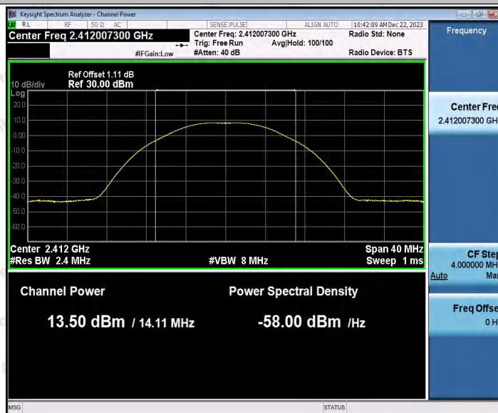
802.11b_Ant2_2412
