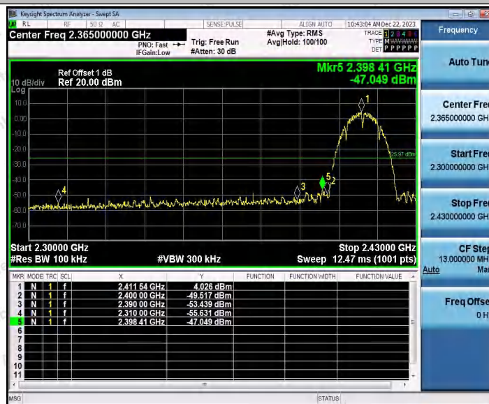
802.11b_Ant2_Low_2412
