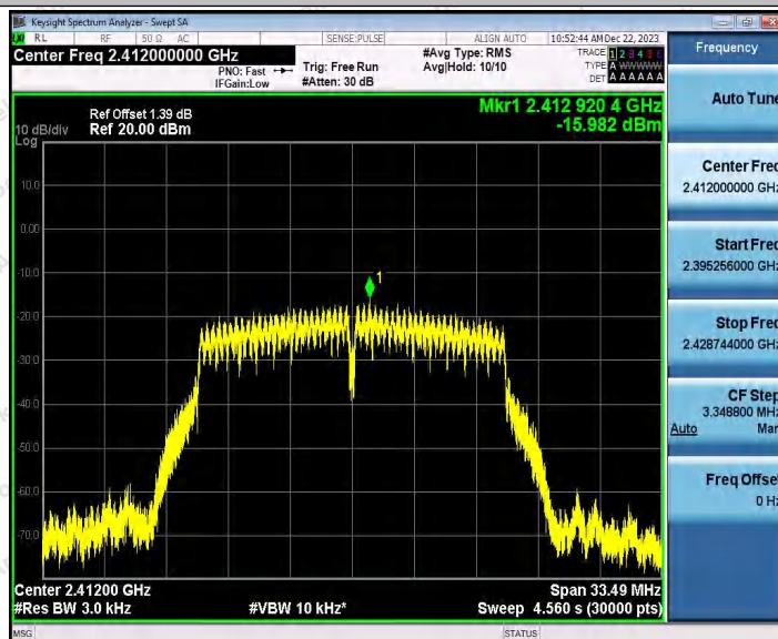
802.11g_Ant2_2412
