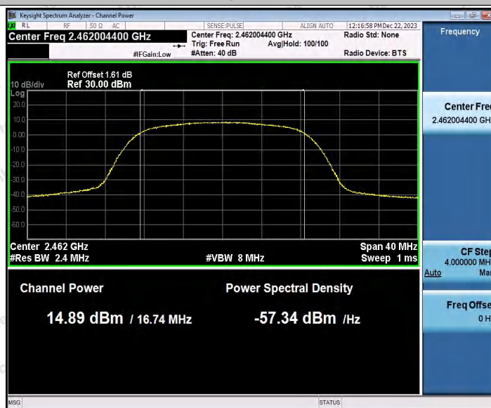
802.11g_Ant2_2462
