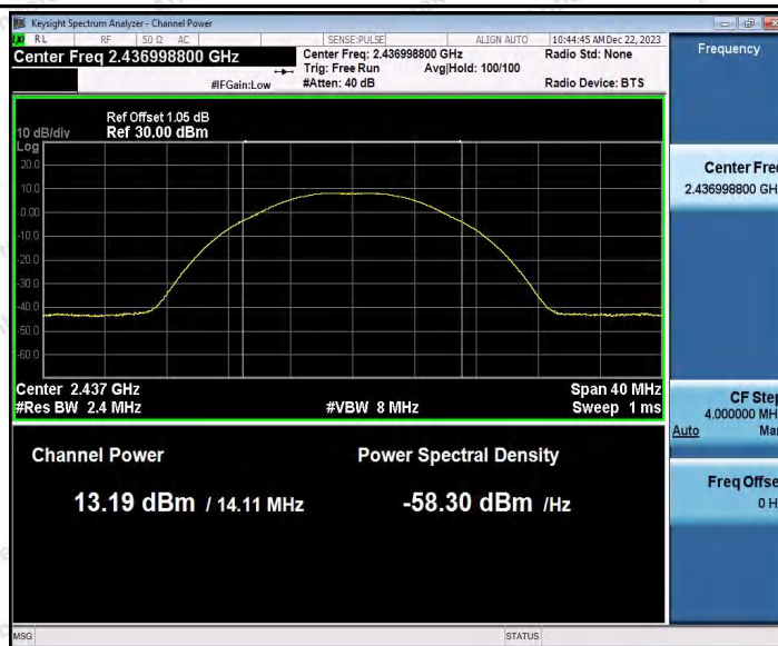
802.11b_Ant2_2437
