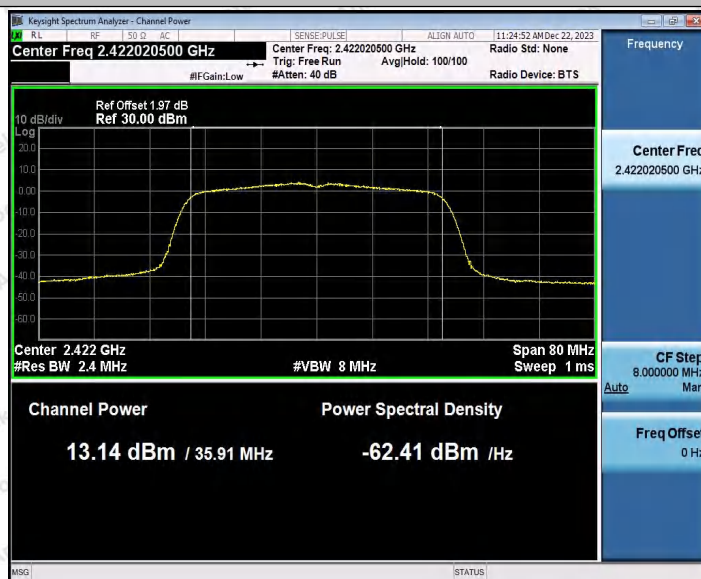
802.11n(HT40)SISO_Ant2_2422
