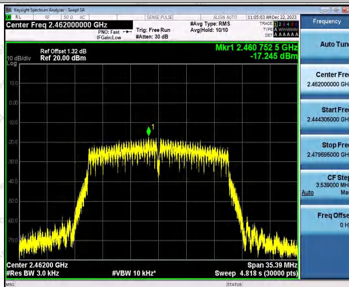
802.11n(HT20)SISO_Ant2_2462
