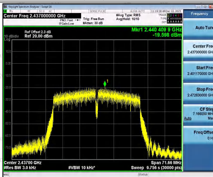
802.11n(HT40)SISO_Ant2_2437
