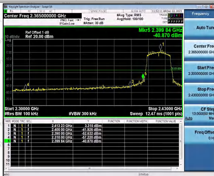
802.11n(HT20)SISO_Ant2_Low_2412
