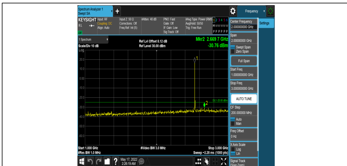
Band7-5MHz-QPSK-21100-1RB#0-Range4:1000~3000MHz
