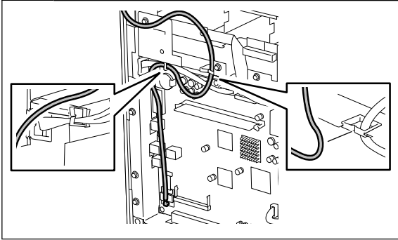
14 WIRE 配線する BRANCHER ANSCHLIESSEN 配线 CONECTAR 配线
