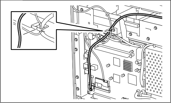
17 WIRE 配線する BRANCHER ANSCHLIESSEN 配线 CONECTAR 配线
