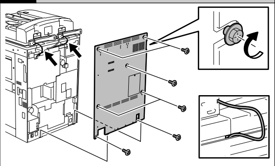
24 INSTALL 取付ける INSTALLER EINSETZEN 装上 INSTALAR 装上
