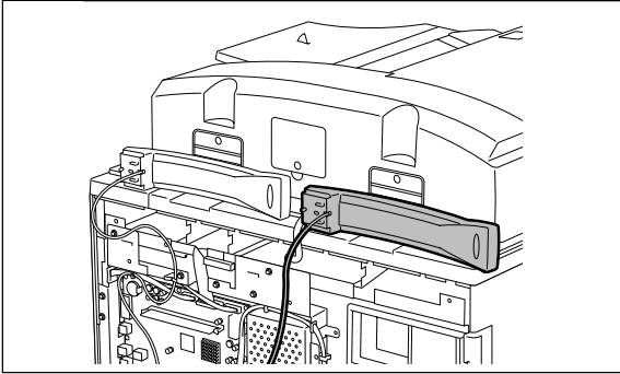
15 PLACE 置く PLACER EINLEGEN 放入 COLOCAR 放入
