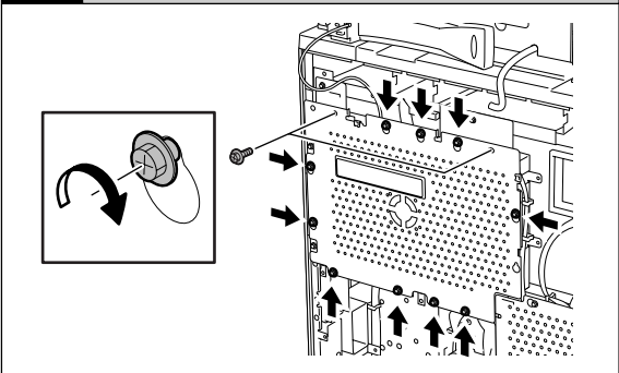
20 INSTALL 取付ける INSTALLER EINSETZEN 装上 INSTALAR 装上
