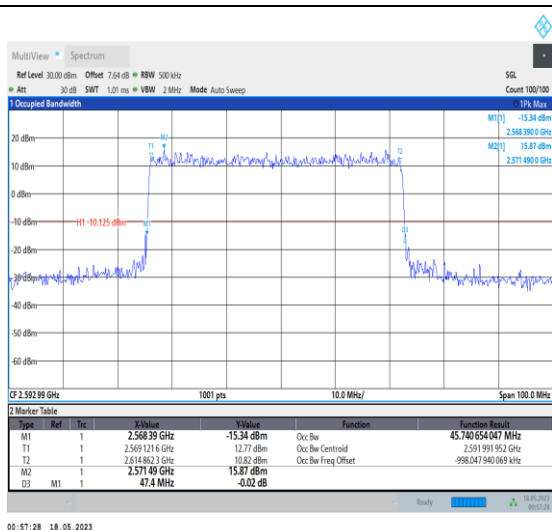
1-N41-PC1-30-50-M-3-DFT-16QAM-Outer_Full-128 @0-Ant0-45.741-47.400-≤50-PASS
