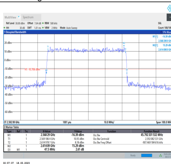
1-N41-PC1-30-50-M-4-DFT-64QAM-Outer_Full-128 @0-Ant0-45.792-47.500-≤50-PASS
