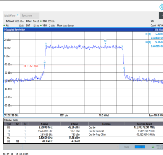
1-N41-PC1-30-50-M-6-CP-QPSK-Outer_Full-133@0 -Ant0-47.37-49.300-≤50-PASS
