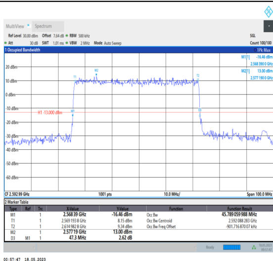
1-N41-PC1-30-50-M-5-DFT-256QAM-Outer_Full-128 @0-Ant0-45.789-47.300-≤50-PASS
