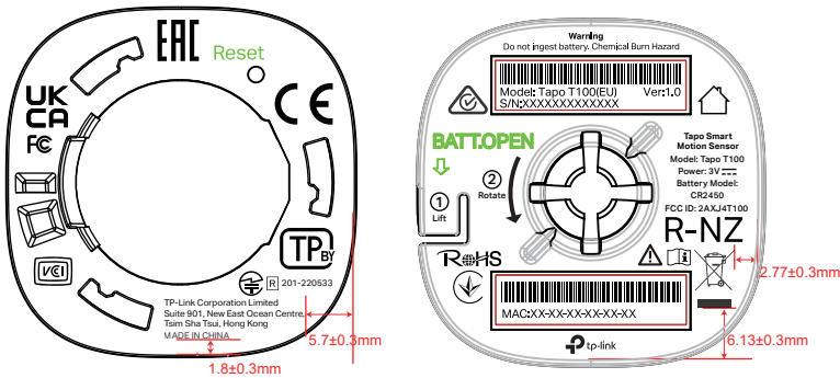
尺寸图
