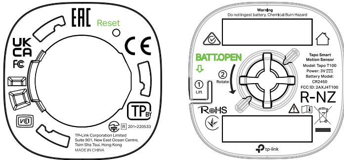
效果图（转曲）
