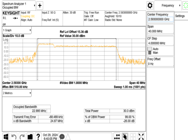
Band41_20MHz+5MHz_QPSK_RB100-0+RB25-0_CH40595+CH40712
