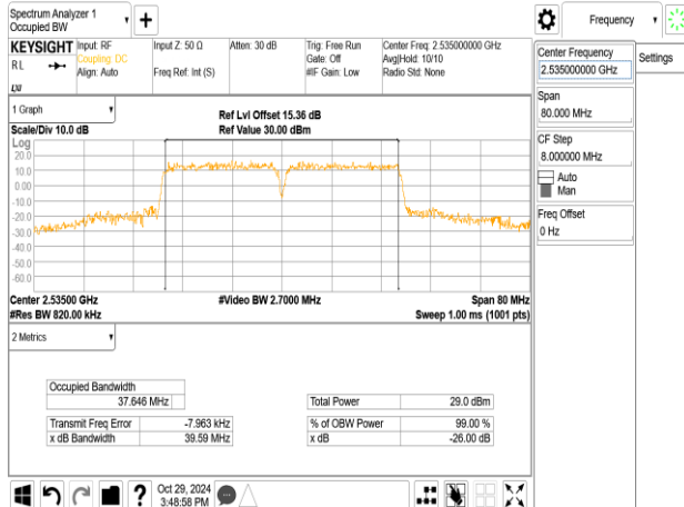
Band7_20MHz+20MHz_16QAM_RB100-0+RB100-0_CH21001+CH21199
