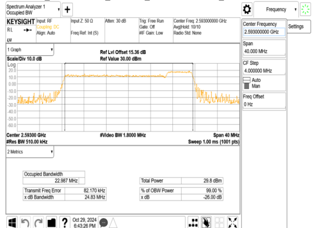
Band41_10MHz+20MHz_QPSK_RB50-0+RB100-0_CH40526+CH40670
