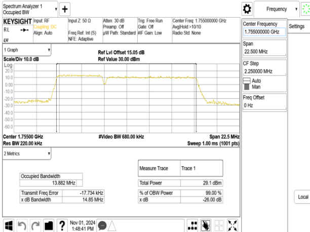
Band66B_10MHz+5MHz_QPSK_RB50-0+RB25-0_CH132397+CH132469
