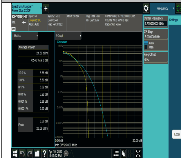
66-66-10MHz-10MHz-QPSK-QPSK-132523-132622-50RB#0-50RB#0-PASS
