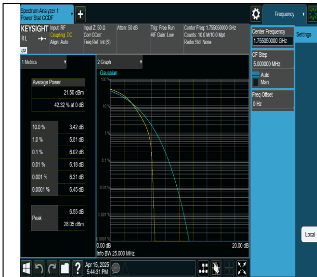
66-66-10MHz-10MHz-QPSK-QPSK-132373-132472-50RB#0-50RB#0-PASS
