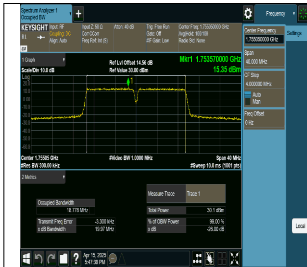
66-66-10MHz-10MHz-QPSK-QPSK-132373-132472-50RB#0-50RB#0-PASS
