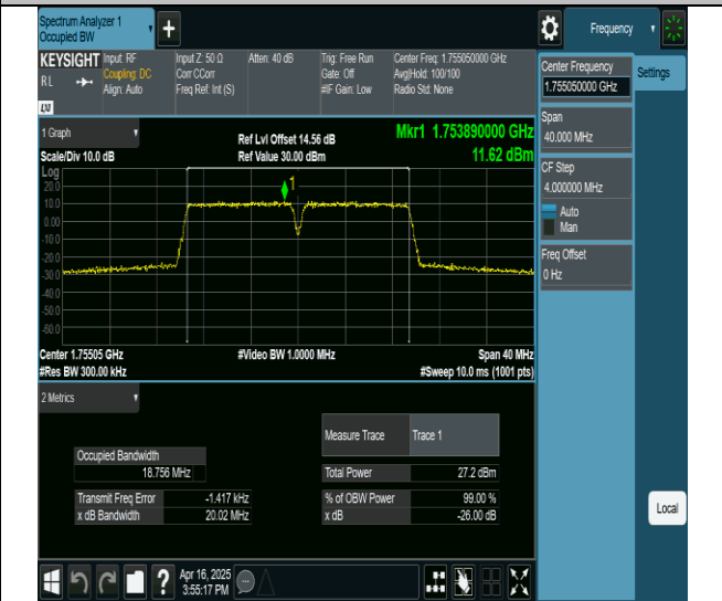
66-66-10MHz-10MHz-256QAM-256QAM-132373-132472-50RB#0-50RB#0-PASS
