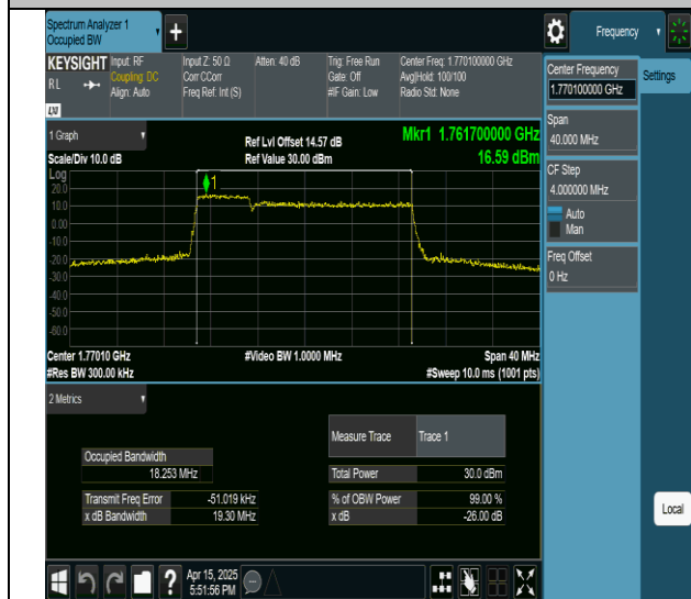
66-66-5MHz-15MHz-QPSK-QPSK-132504-132597-25RB#0- 75RB#0-PASS
