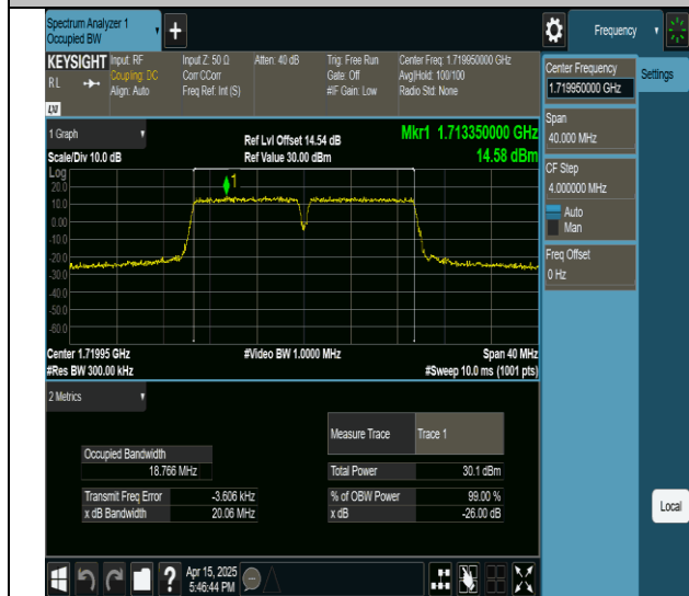
66-66-10MHz-10MHz-QPSK-QPSK-132022-132121-50RB#0-50RB#0-PASS
