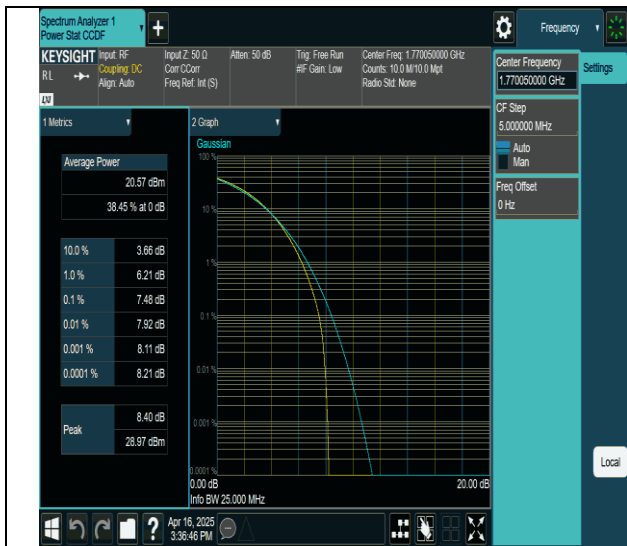
66-66-10MHz-10MHz-64QAM-64QAM-132523-132622-50RB#0- 50RB#0-PASS
