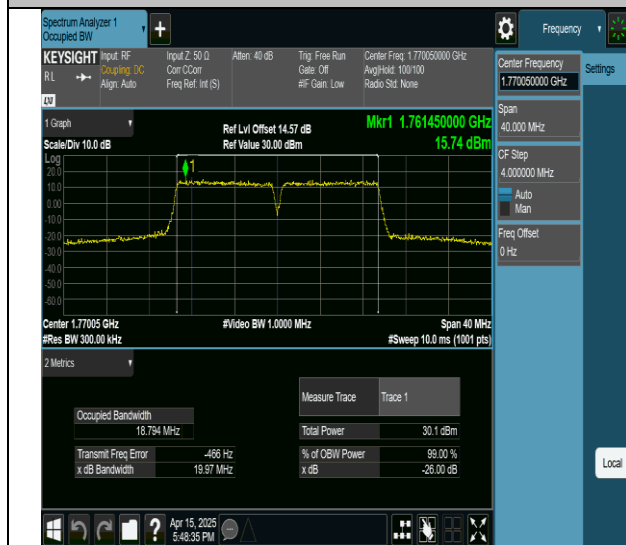
66-66-10MHz-10MHz-QPSK-QPSK-132523-132622-50RB#0-50RB#0-PASS
