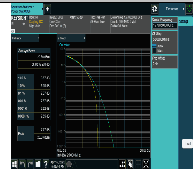
66-66-10MHz-10MHz-16QAM-16QAM-132523-132622-50RB#0-50RB#0-PASS
