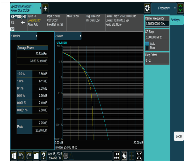
66-66-10MHz-10MHz-16QAM-16QAM-132373-132472-50RB#0-50RB#0-PASS
