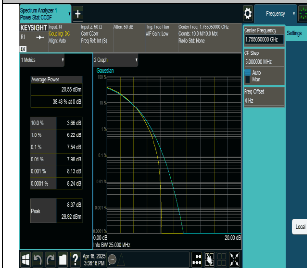
66-66-10MHz-10MHz-64QAM-64QAM-132373-132472-50RB#0-50RB#0-PASS
