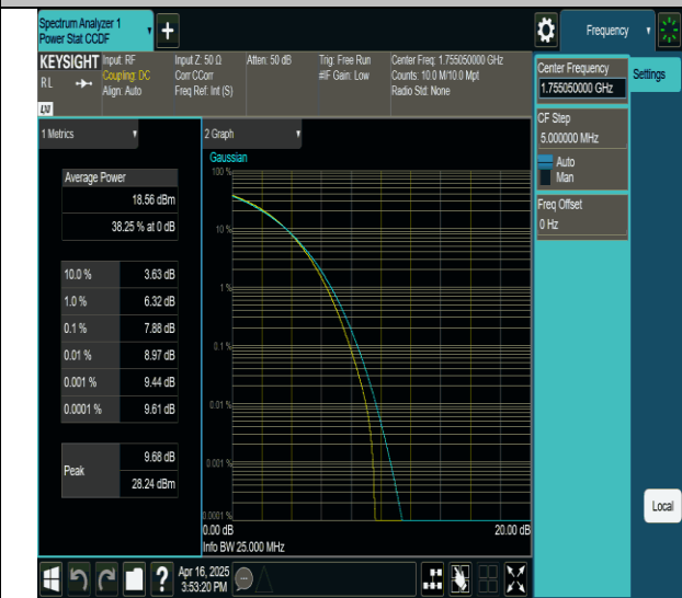
66-66-10MHz-10MHz-256QAM-256QAM-132373-132472-50RB#0-50RB#0-PASS
