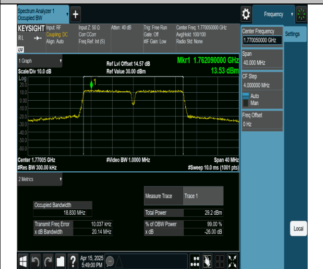
66-66-10MHz-10MHz-16QAM-16QAM-132523-132622-50RB#0-50RB#0-PASS
