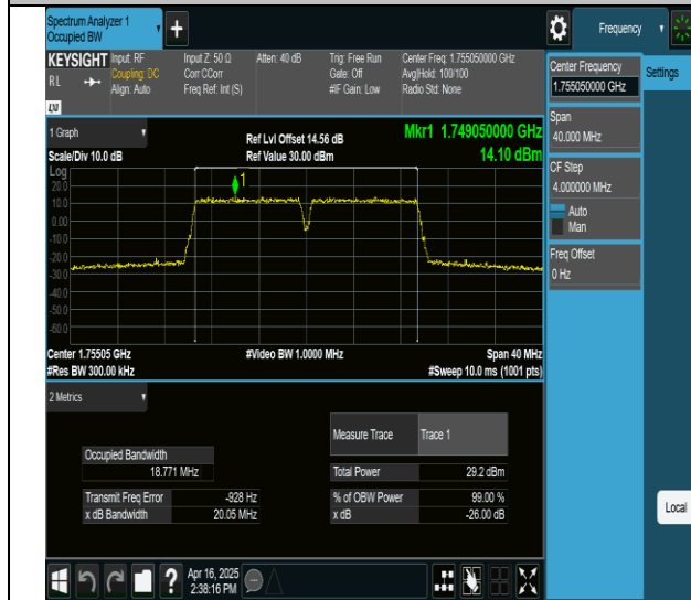
66-66-10MHz-10MHz-64QAM-64QAM-132373-132472-50RB#0-50RB#0-PASS
