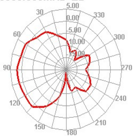
5850.000MHz E2
