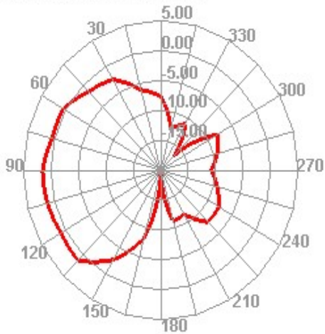
5800.000MHz E2
