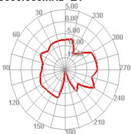
5800.000MHz E1
