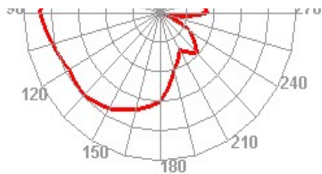
5850.000MHz E2
