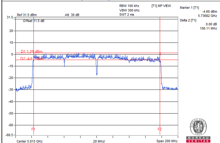
802.11be (EHT160) / Chain 2 : CH 163
