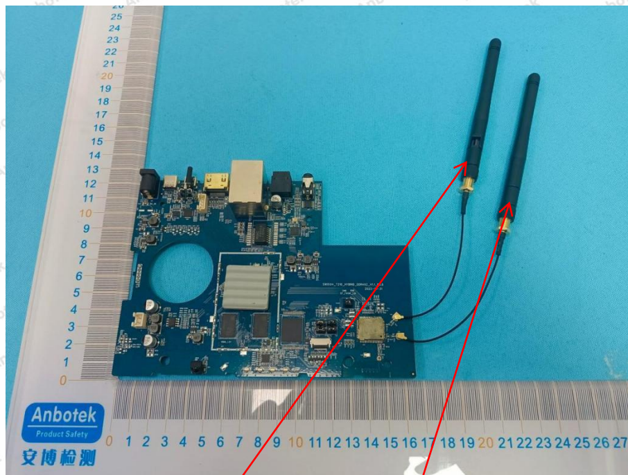
BT&WIFI ANT1
