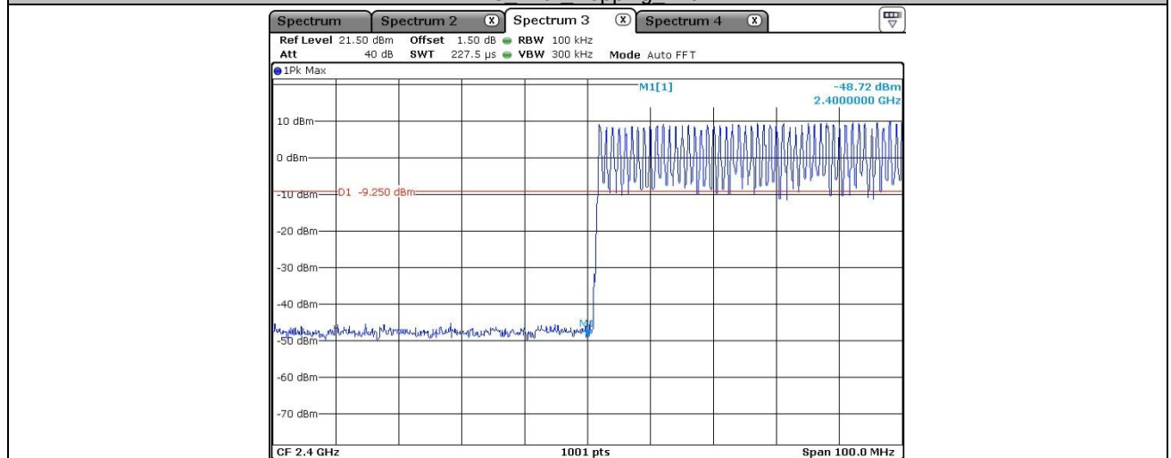
DH5 Ant1 Hopping 2402
